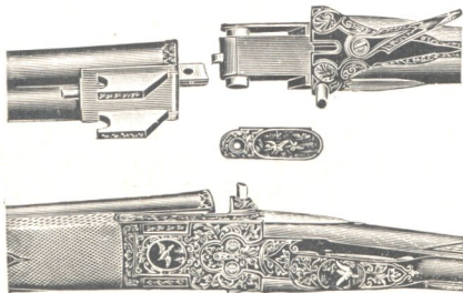
Simson-Jäger-Verschluß zerlegt und von unten gesehen.
