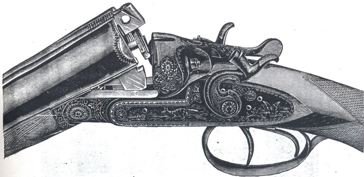
Фабрики А. Франкотт и К о , въ Льежѣ.
