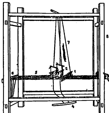
საქსოვი დაზგა: 1. სავარცხელი, 2. „ზინგი“, 3. ლირე, 4. საფეხური, 5. ქსელი, 6. „ზვიცელი“, 7. თოკი, 8. ჩარჩო.
