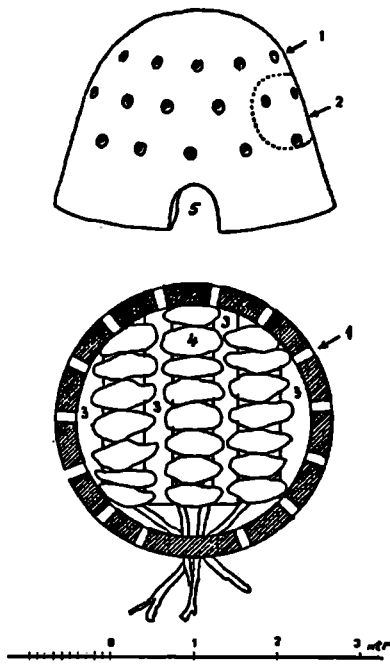
ქურის ნაწილები: 1. საპაერო ზვრელი - „თოლი“, 2. ჭურჭლის ჩასაწყობი, 3. ტახტი, 4. რიყის ქვები, 5. ღუმელი.
