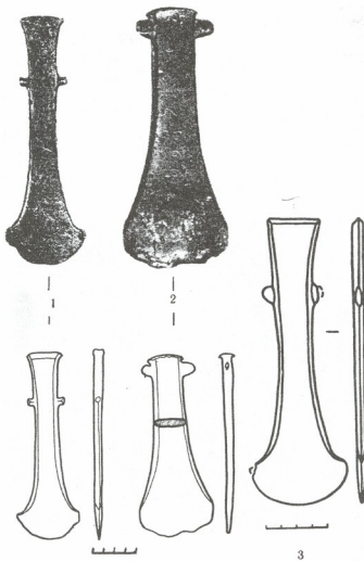
ბრტყელი ცული ბრინჯაოსი. აღმოჩენილია უშგულში. ინახება უშგულის მუზეუმში. სიმაღლე 18,0 სმ. სისქე - 0,5 სმ., პირის ფართი - 6,5 სმ.
