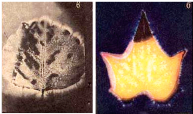
კირლიანის ფოტოეფექტი
