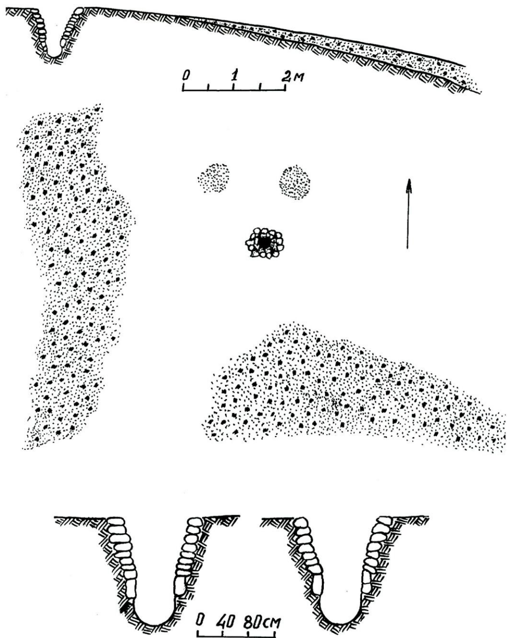
სურ. 7. რკინისადნობი სახელოსნო „ჯიხანჯური II“,
