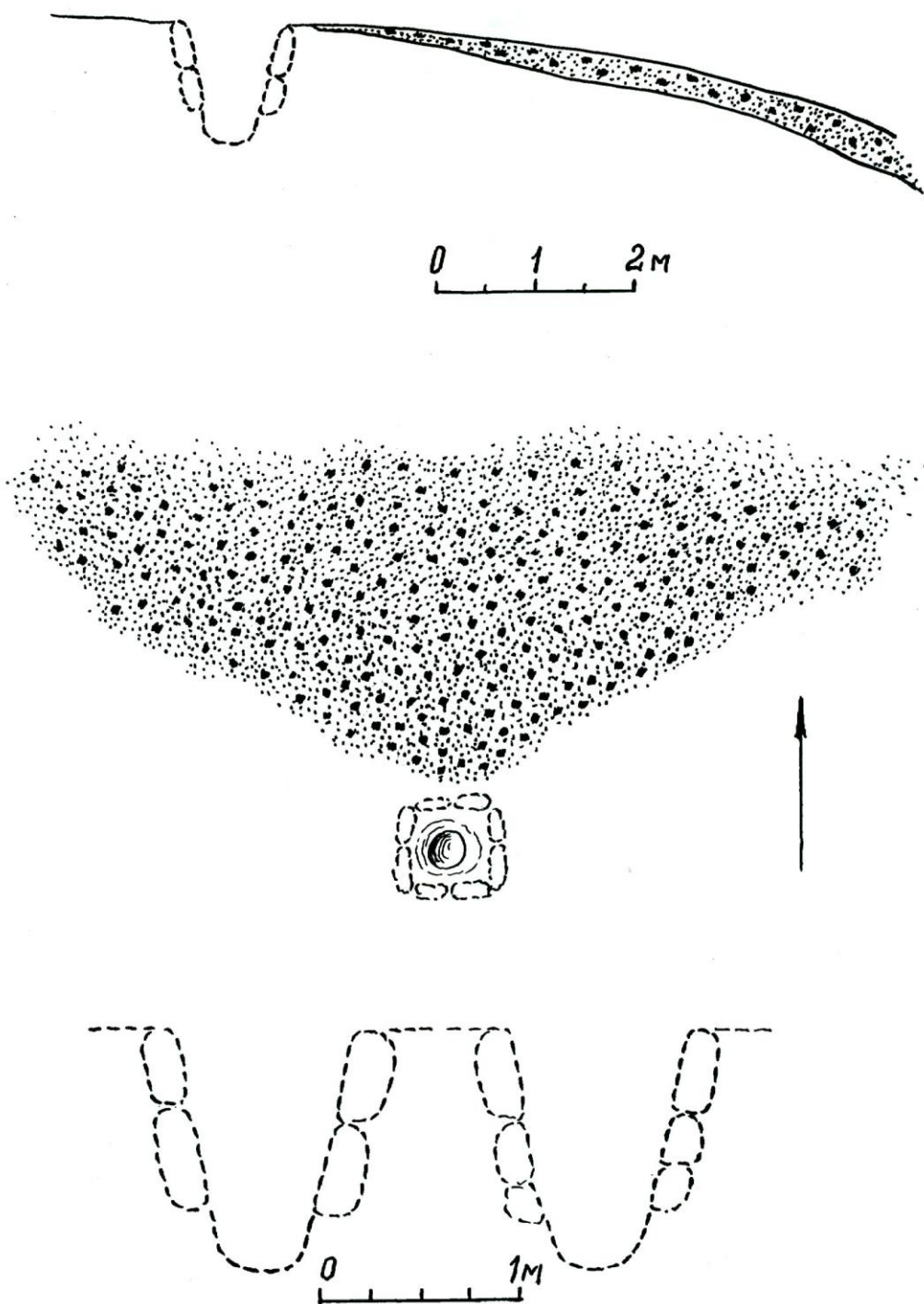
სურ. 6. რკინისსადნობი სახელოსნო „ჯიხანჯური I.3“,
