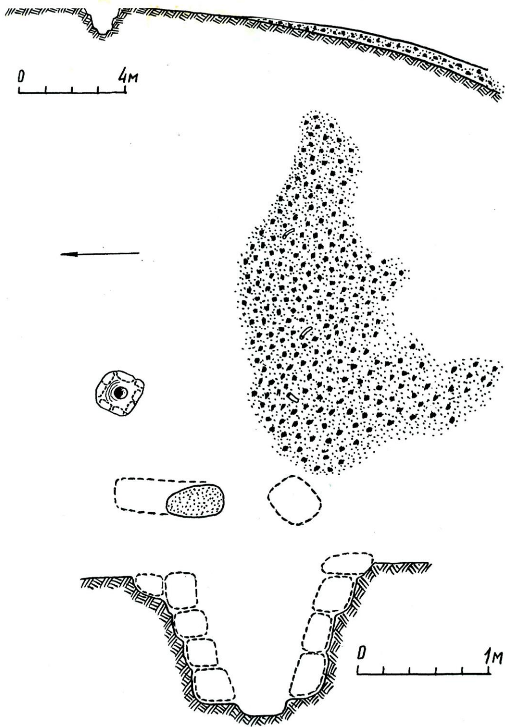
სურ. 13. რკინისაღნობი სახელოსნო „გეგბლაური I“
