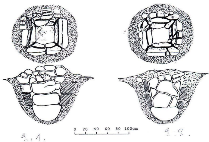
სურ. 19. რკინისადავარი სახელოსნო „ჩაისუბანი I“
