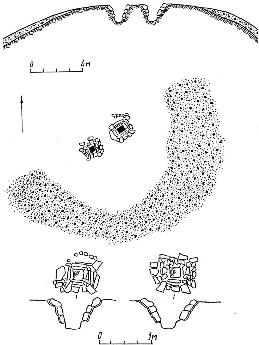
სურ. 10. რკინისაღნოზი სახელოსნო „ლეღვა I.1“ და „ლეღვა I.2“
