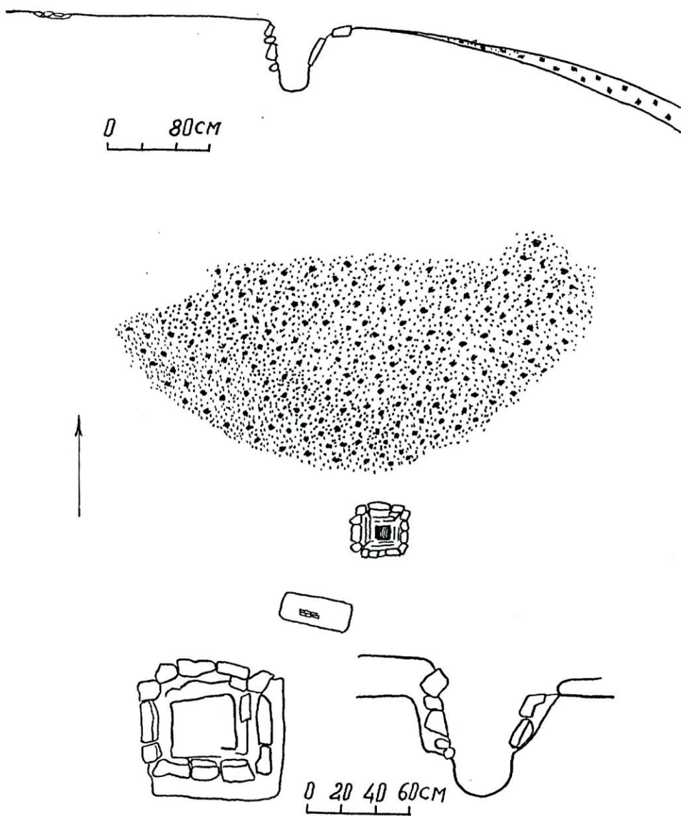
სურ. 9. რკინისადნობი სახელოსნო „გიხანჯური IV“,
