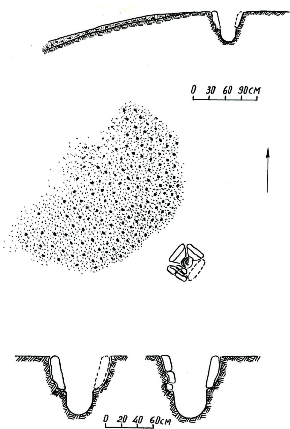
სურ. 5. რკინისსადნობი სახელოსნო „ჯიხანჯური I.2“,
