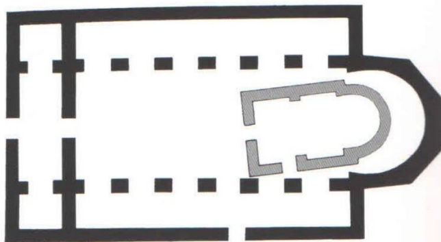
5. ციხისძირის ბაზილიკისა და დარბაზული ეკლესიის გეგმა
