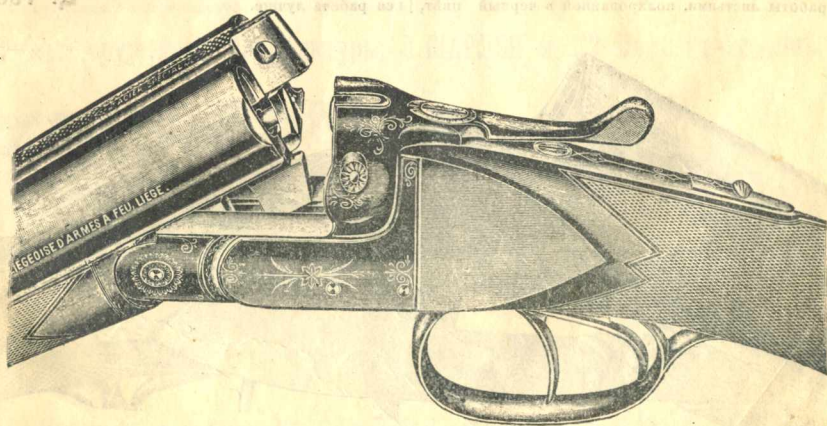
№ 17. Ружье безкурковое Льежской Мануфактуры, с эжектором.
