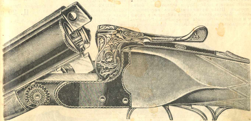
№ 162. Безкурковое ружье Национальной фабрики, с эжектором усовершенствованной системы Голланда.
