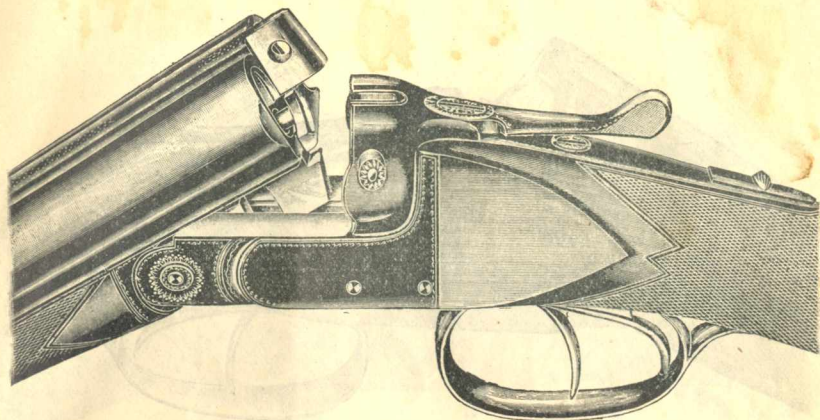
№ 16. Ружье безкурковое Льежской Мануфактуры.
