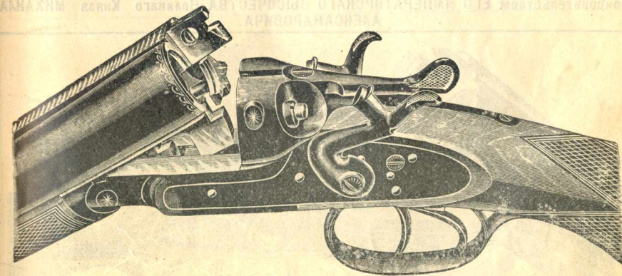
№ 101. Ружье фабрики А. Бертрана и К о .
