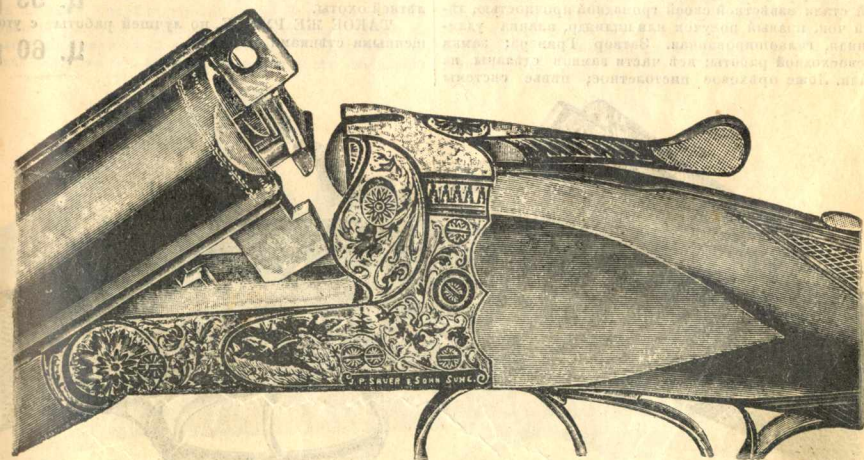
№ 140. Безкурковое ружье I. П. Зауэра и Сына с эжектором. Марка „Мейстерверк“, максимальный бой, „Höchstleistung“.
