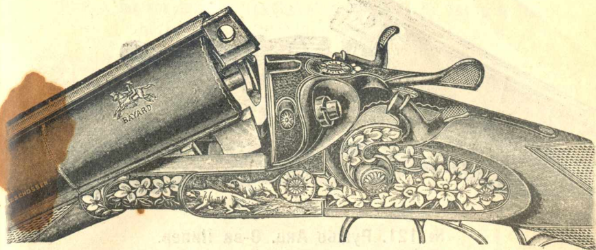
№ 119. Ружье Акц. О-ва Пипер.
