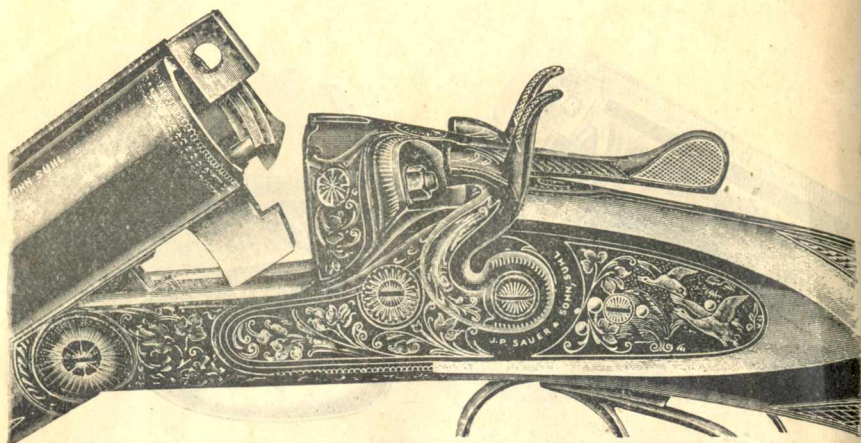
№ 129. Ружье фабрики I. П. Зауэра и Сына.
