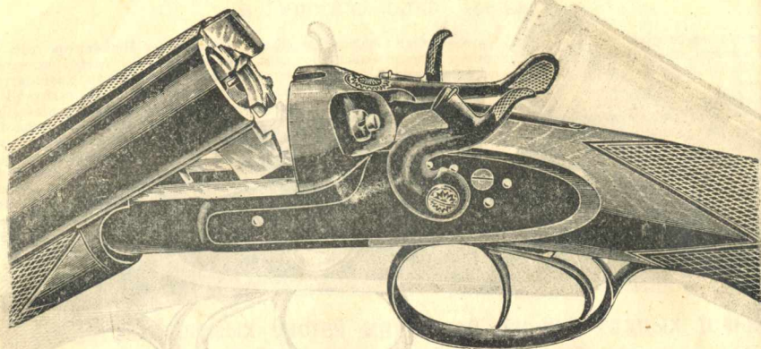
№ 155. Ружье „Прима“ Национальной фабрики военного оружія.
