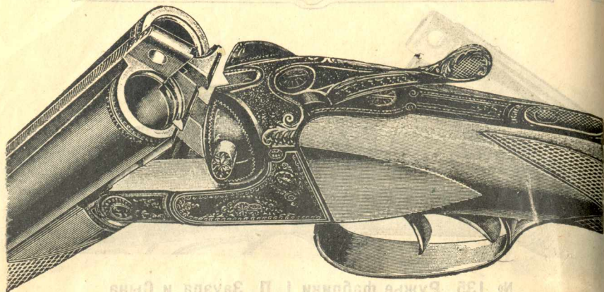
№ 137. Садочного типа безкурковое ружье фабрики I. П. Зауэра и Сына.
