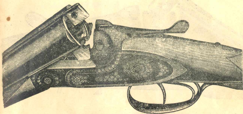
№ 60. Садовое ружье фабрики Франкотта системы Энсон и Дилей, безкурковое.
