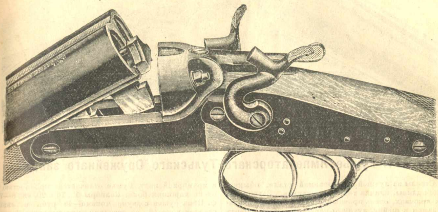
№ 169. Ружье Императорскаго Тульскаго Оружейнаго завода.
