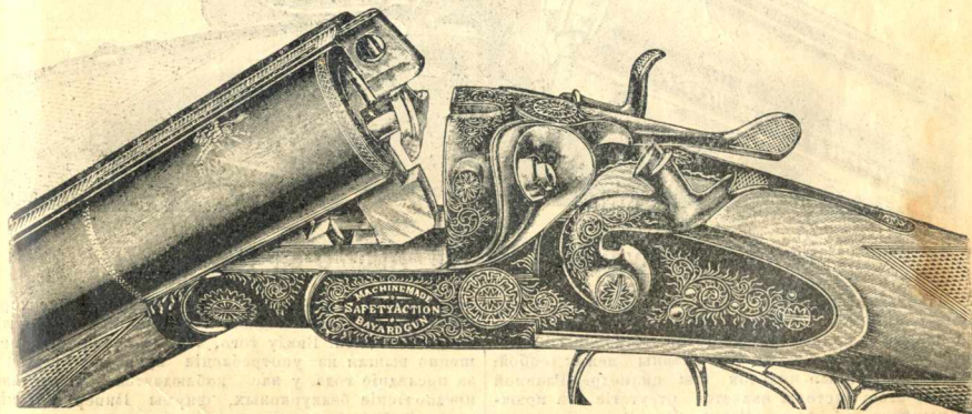
№ 120. Садочнаго типа ружье Акц. О-ва Пипер марки „Діана“.
