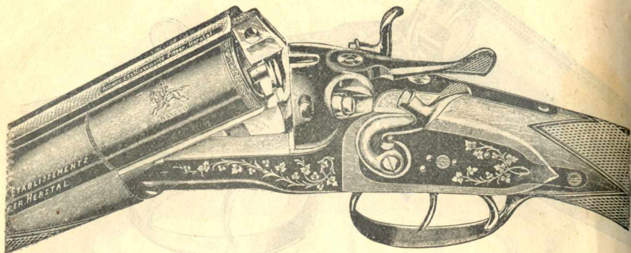
№ 113. Ружье Акц. О-ва Пипер в Льежѣ.
