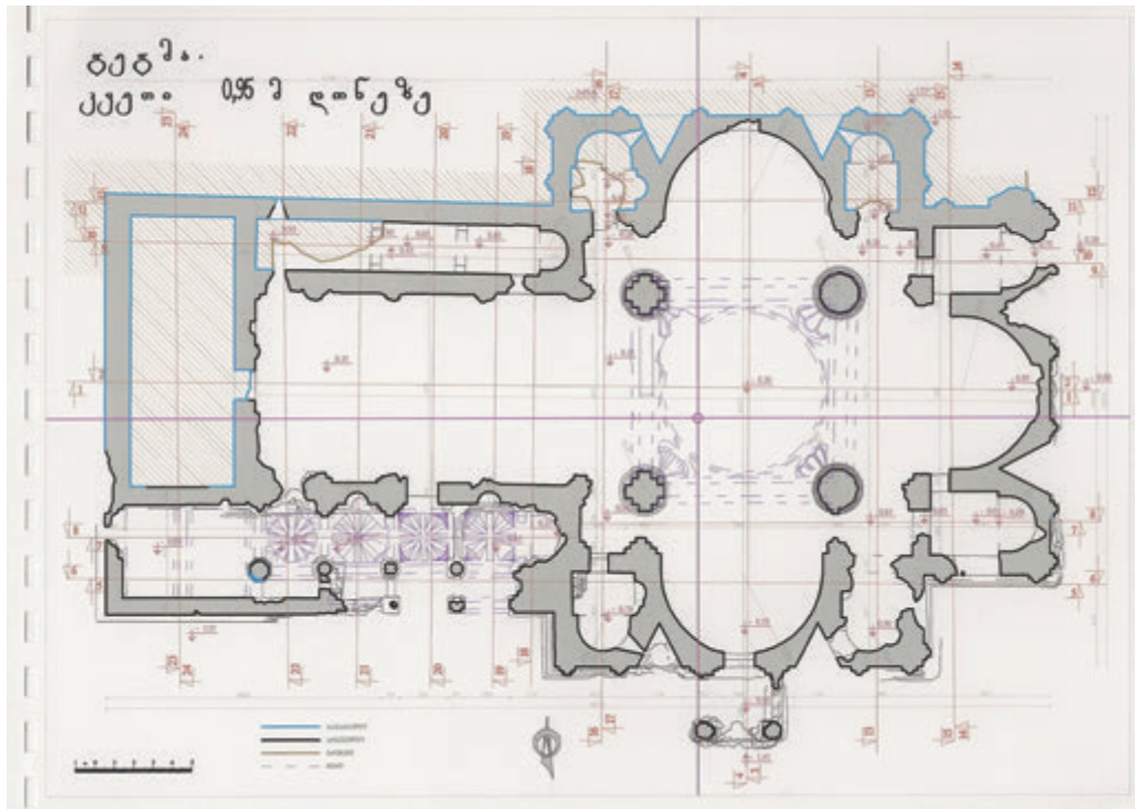
ოშკი, გეგმა, ვ. გრემელაშვილის ანაზობი
