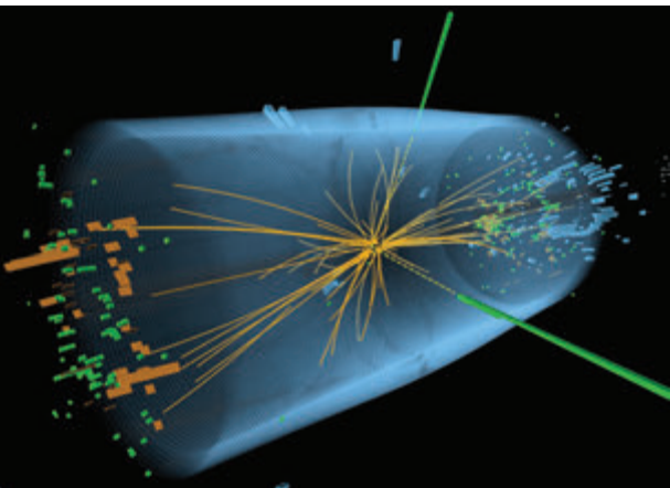
პიესის ბოზონის აღმოჩენის სქემატური გამოსახულება
