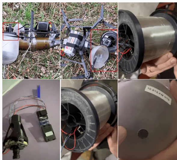
რუსულ FPV დრონზე დამაგრებული საკომუნიკაციო სისტემები, 2024 წლის მარტი ფოტო: Serhii Flash, წყარო: mil.in.ua
