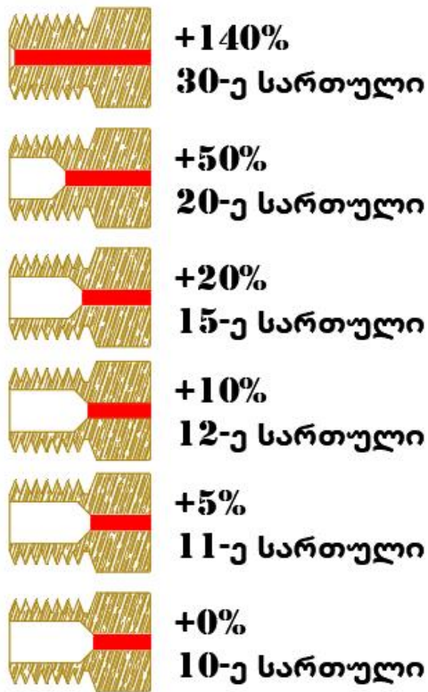
ნახ36. მაღლივ შენობაში 10-ე სართულის შემდეგ სიმაღლეზე ნაცმის ბუნებრივი აირის სადინარის (წითლად) სიგრძის დამოკიდებულება % ში, ჰიდროსტატიკური წნევის ზრდის მიხედვით, დარს-ვეისბახის დაბალი წნევის ქსელში, წნევის ვარდნის ფორმულის თანახმად.
