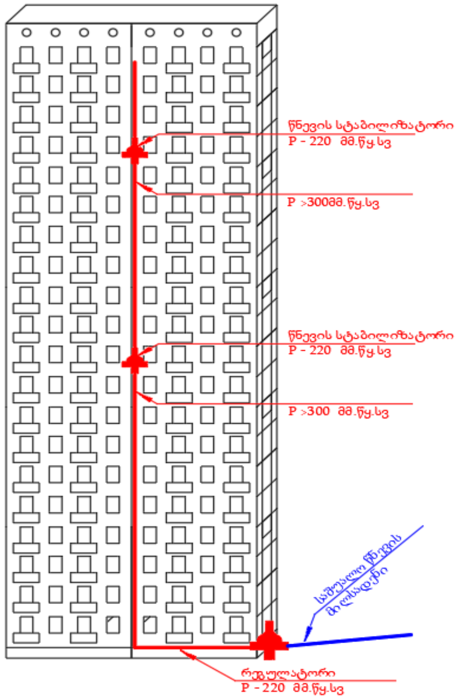
ნახ. 38 მაღლივ საცხოვრებელ შენობაში, სიმაღლის მიხედვით გაზის ჰიდროსტატიკური წნევის მატების სტაბილიზაციის მოდელი
