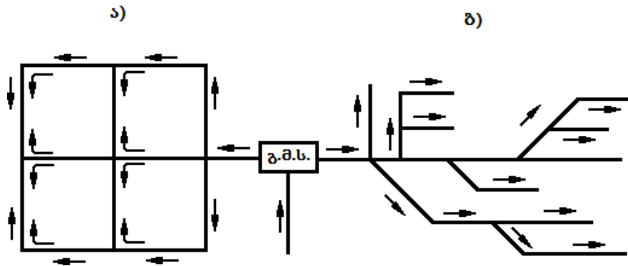
ნახ. 1 გაზმომარაგების ა. რგოლური ქსელის სქემა; ბ. ჩიხური ქსელის სქემა.
