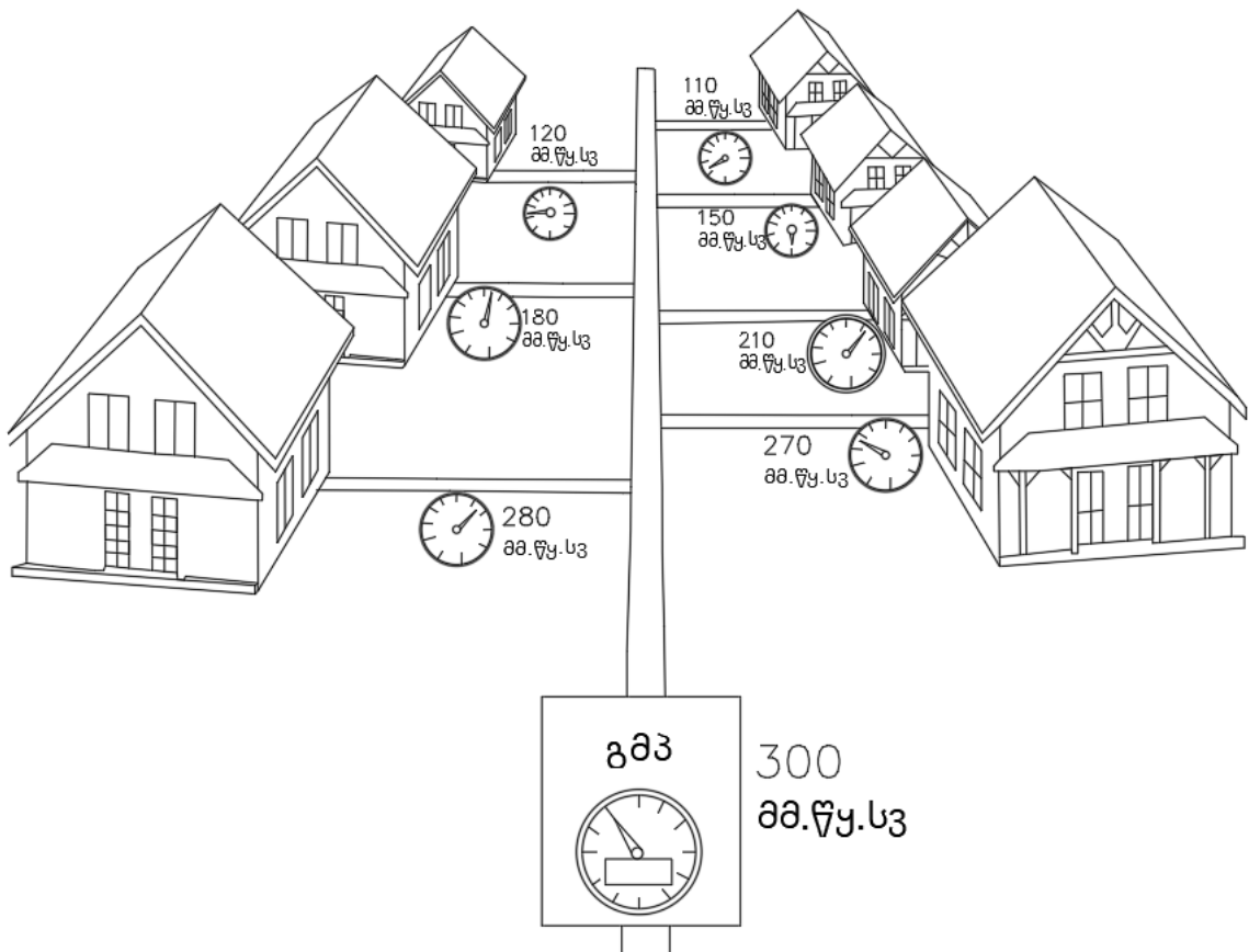
ნახ. 31 არსებული ნორმებით დადგენილი დაბალი წნევის გაზის ქსელის სქემა
