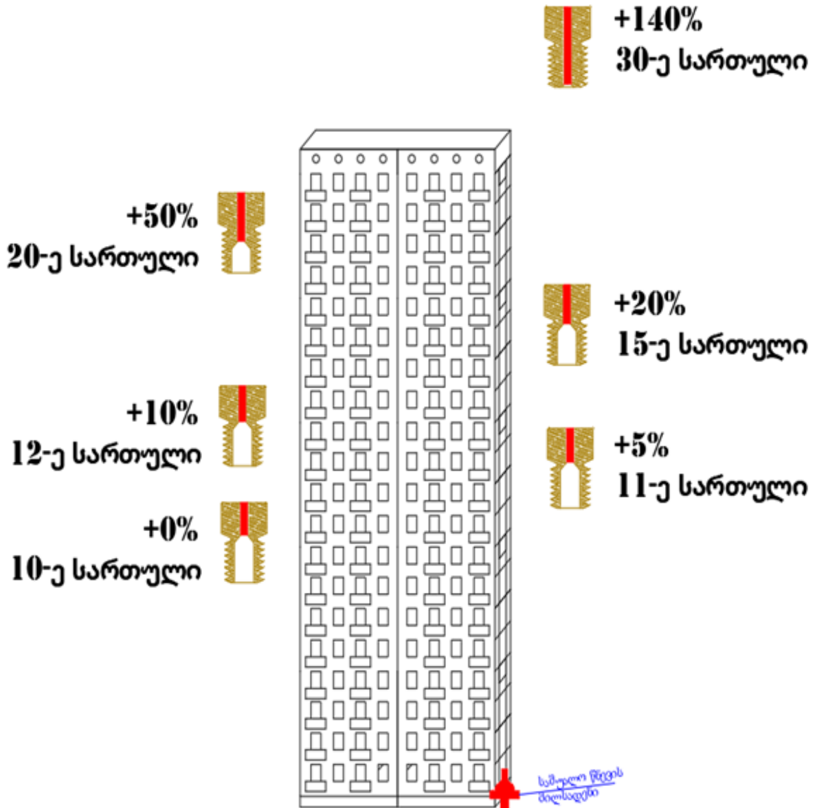
ნახ37. სართულების მიხედვით, ნომინალურ წნევასთან მიახლოებისთვის გაზდანადგარში ნაცმის შერჩევის მოდელი
