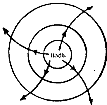
ნახ. 12.2.5. ანტიციკლონი
