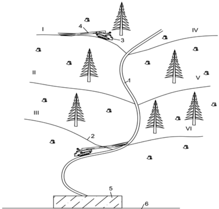
ნახ. 1. ტექნოლოგიური სქემა № 1ა.
