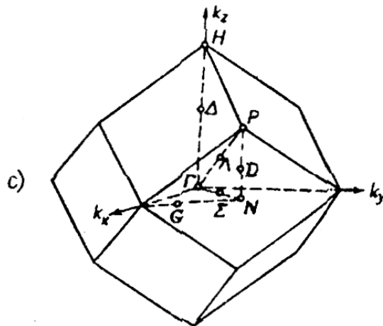
Рис. 4. Первые зоны Бриллюэна типичных металлических кристаллических решеток
