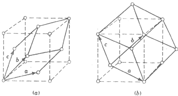
Рис. 1. Примитивные ячейки кубической грани- (а) и объемно- (б) центрированной решетки с примитивными трансляционными векторами \vec{a}, \vec{b}, \vec{c} (т.е. векторами \vec{a}_1, \vec{a}_2, \vec{a}_3 из уравнения (1))
