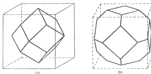
Рис. 3. Элементарные симметричные ячейки (атомные ячейки Вигнер-Зейца) для кубической гранецентрированной решетки (а) и кубической объемноцентрированной решетки. Узловые точки находятся в центре представленных ячеек и далее в центре граней (а) или вершин куба
