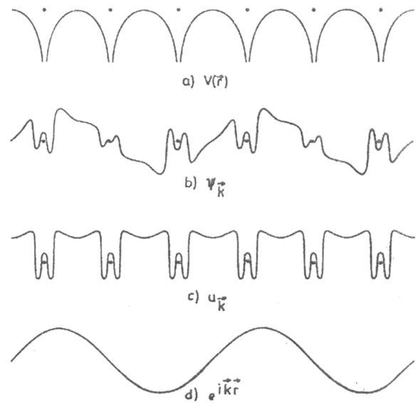
Рис. 2. Схематическое изображение волновых функций электрона в идеальном кристалле: (а) - потенциал вдоль ряда ионов; (б) - реальная часть волновой функции \Psi_{n\vec{k}}(\vec{r}) , которая по (6) является произведением функции u_{n\vec{k}}(\vec{r}) ; (с) - кривая (б) и плоской волны e^{i\vec{k}\vec{r}} , чья реальная часть - кривая (д) согласно [1]
