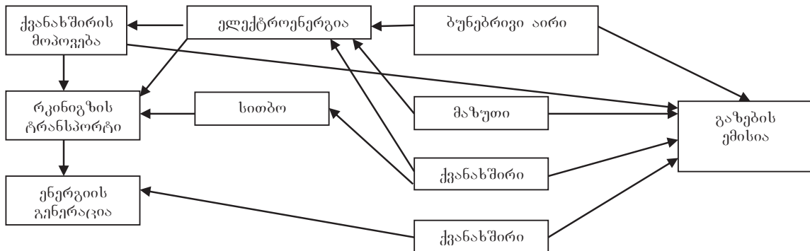
ნახ. 1. ნახშირორჟანგის ემისიის მაჩვენებლის გაანგარიშების სქემა ქვანახშირის წვისას
