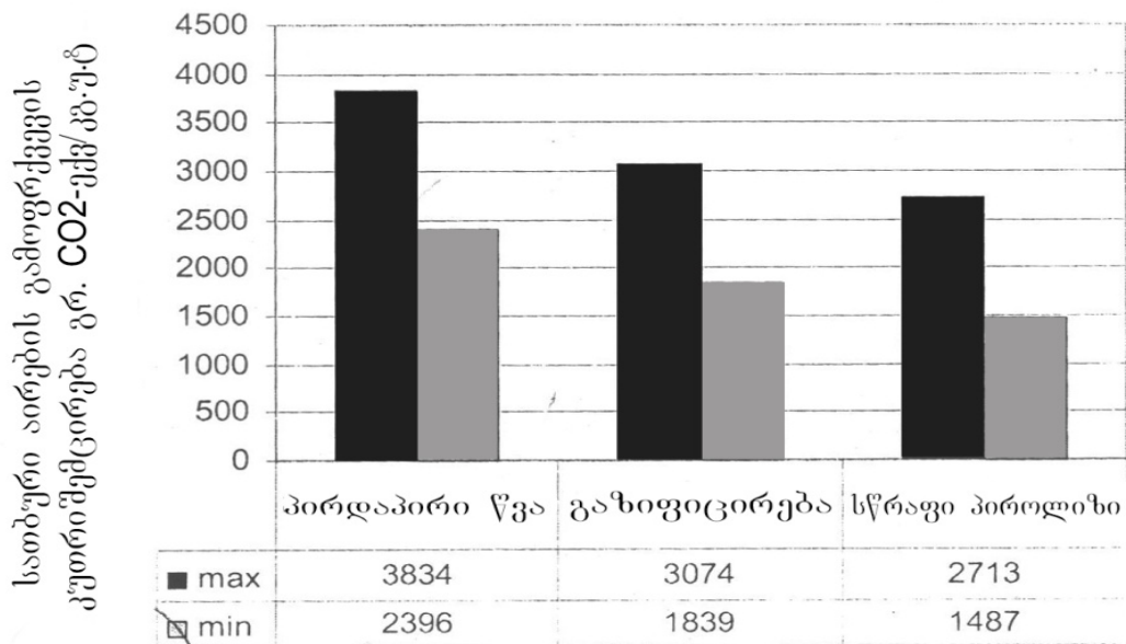
ნახ. 3 სათბური გაზების შემცირების კუთრი მნიშვნელობა სათბური და ელექტრული ენერჯიის კომბინირებული გამოიმუშავებისას
