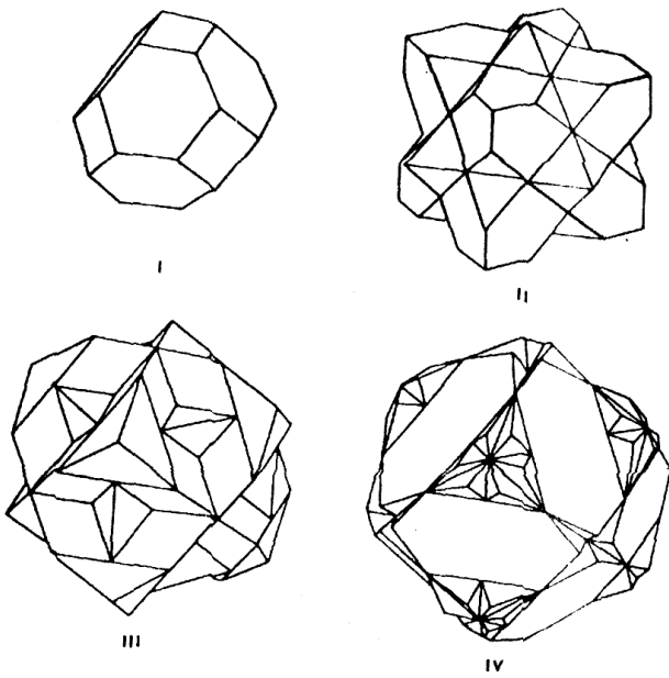
Рис. 5. Граничные поверхности первых четырех зон Бриллюэна кубической объемноцентрированной решетки
