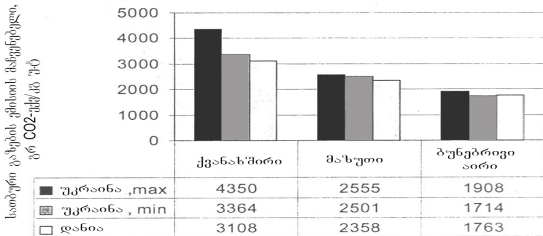
ნახ.2 წიაღისეული სათბობის ემისიის მაჩვენებლები
