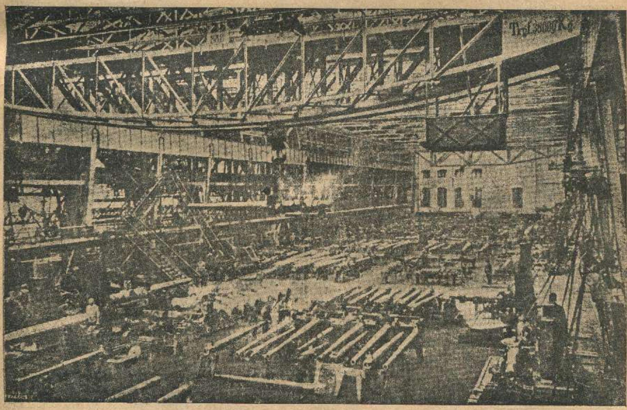
ერთ-ერთი სახელოსნო კრუპის ზარბაზნების ქარხანაში (გერმანიის ჰესენში), სადა მუშაობდა „კატარა“ ზარბაზნები.
