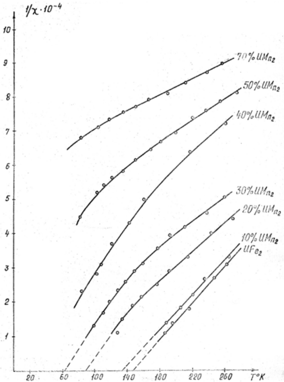
ნახ. 4. კუთრი ამთვისებლობის შებრუნებული სიდიდის ტემპერატურული დამოკიდებულება UMn_2 - UFe_2 სისტემის ყველა ნიმუშისთვის
