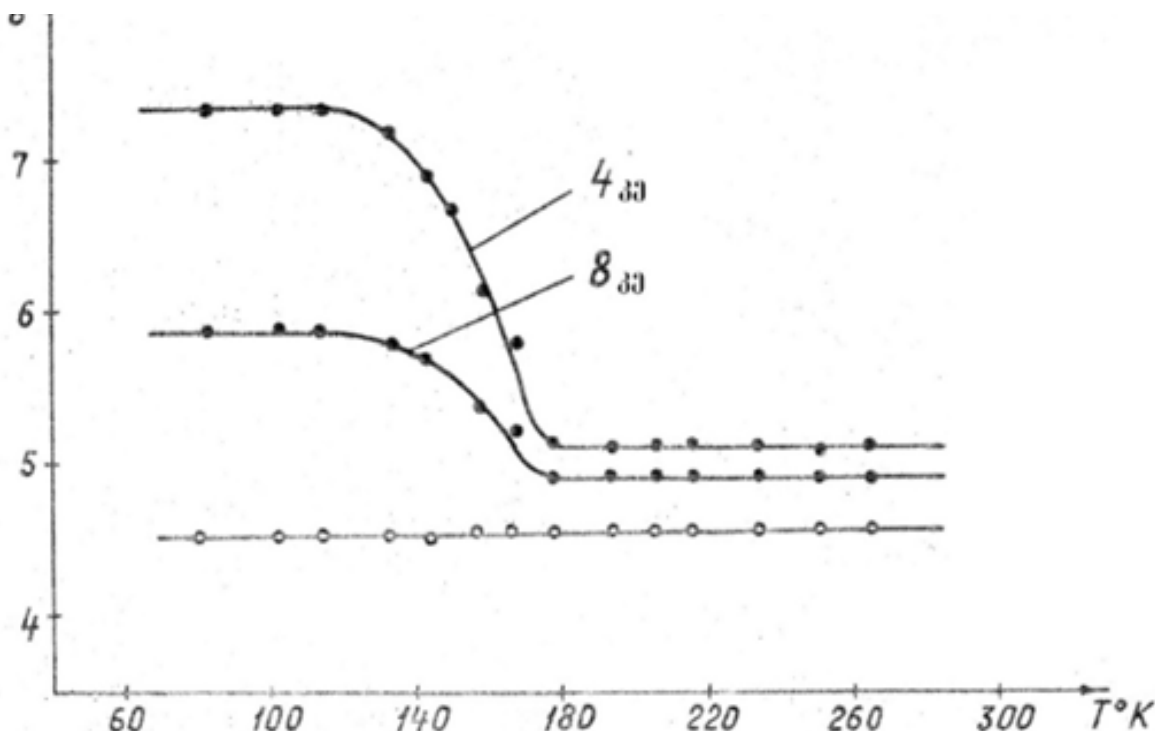
ნახ. 2. UMn_2 ნიმუშის კუთრი ამთვისებლობის ტემპერატურული დამოკიდებულება მრუდი ---0--- ფერომაგნიტური მინარევების გათვალისწინებით
