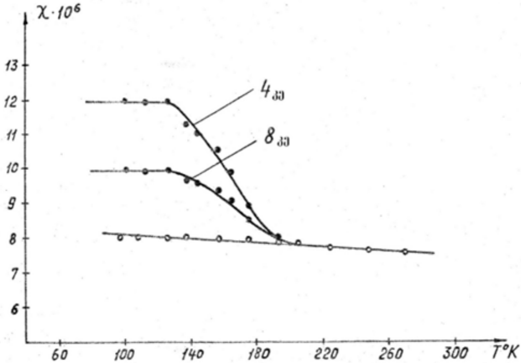
ნახ. 3. 90% UMn_2 - 10% UFe_2 ნიმუშის კუთრი ამთვისებლობის ტემპერატურული დამოკიდებულება (მრუდი ---0--- ფერომაგნიტური მინარევების გათვალისწინებით)
