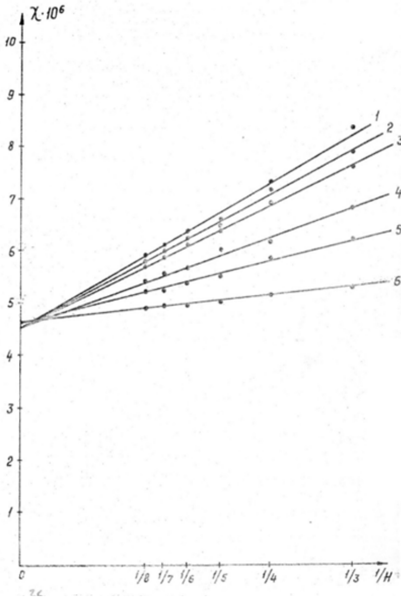
ნახ. 1. UMn_2 ნიმუშის კუთრი ამთვისებლობის ველზე დამოკიდებულება
