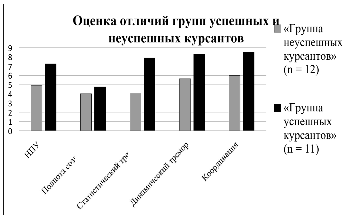
Рис. 3. Оценка достоверности отличий групп успешных и неуспешных курсантов
