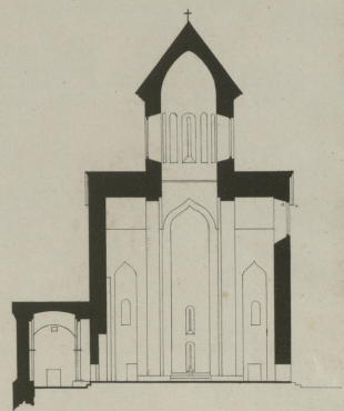
Profil, d'après la ligne N 1.
