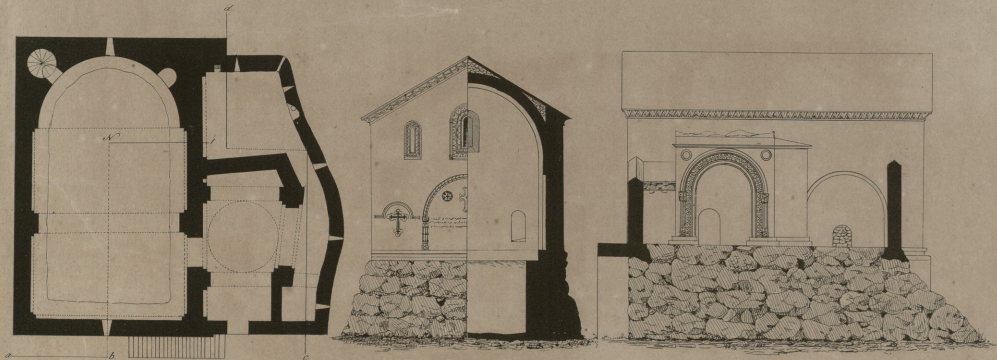
Vue horizontale d'après la ligne a. b.
