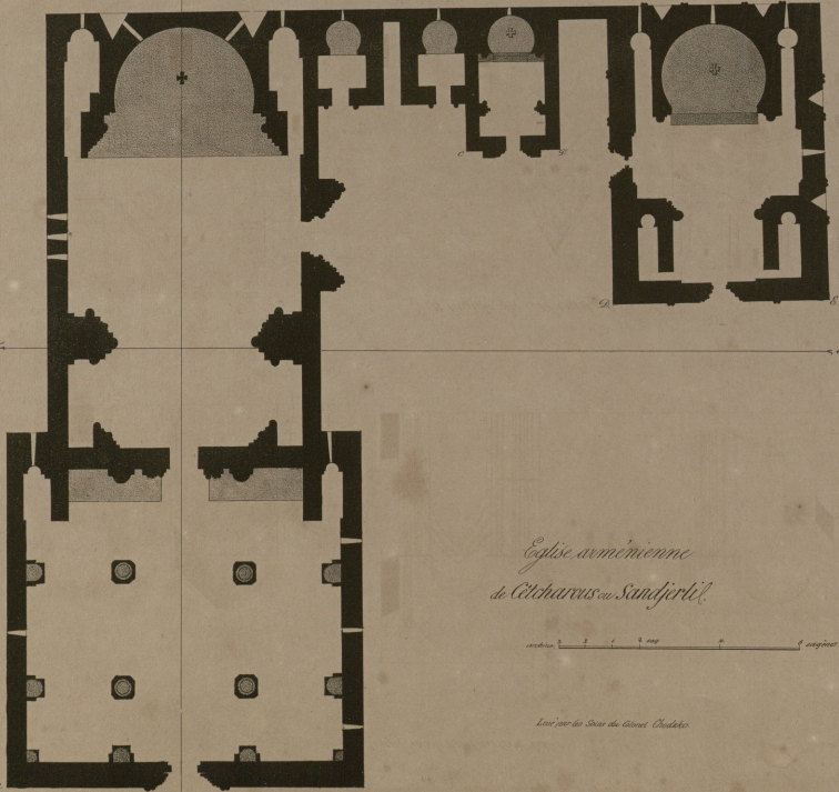
C. Plan général.
