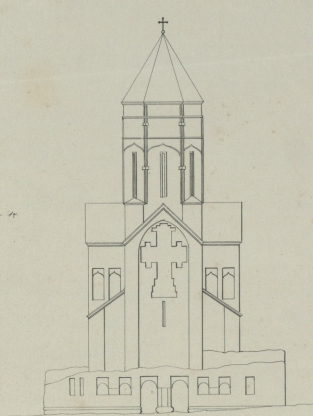
Église d'après la coupe a b
