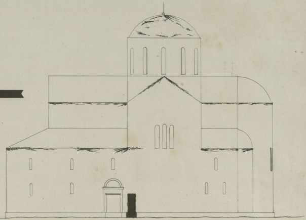
Façade méridionale, d'après la ligne a b.
