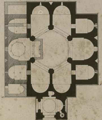
A. Plan de l'église.
