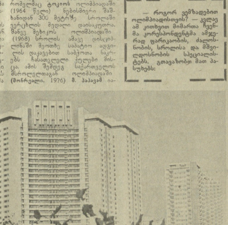
საპროფიტოლოგიის საკითხები...
