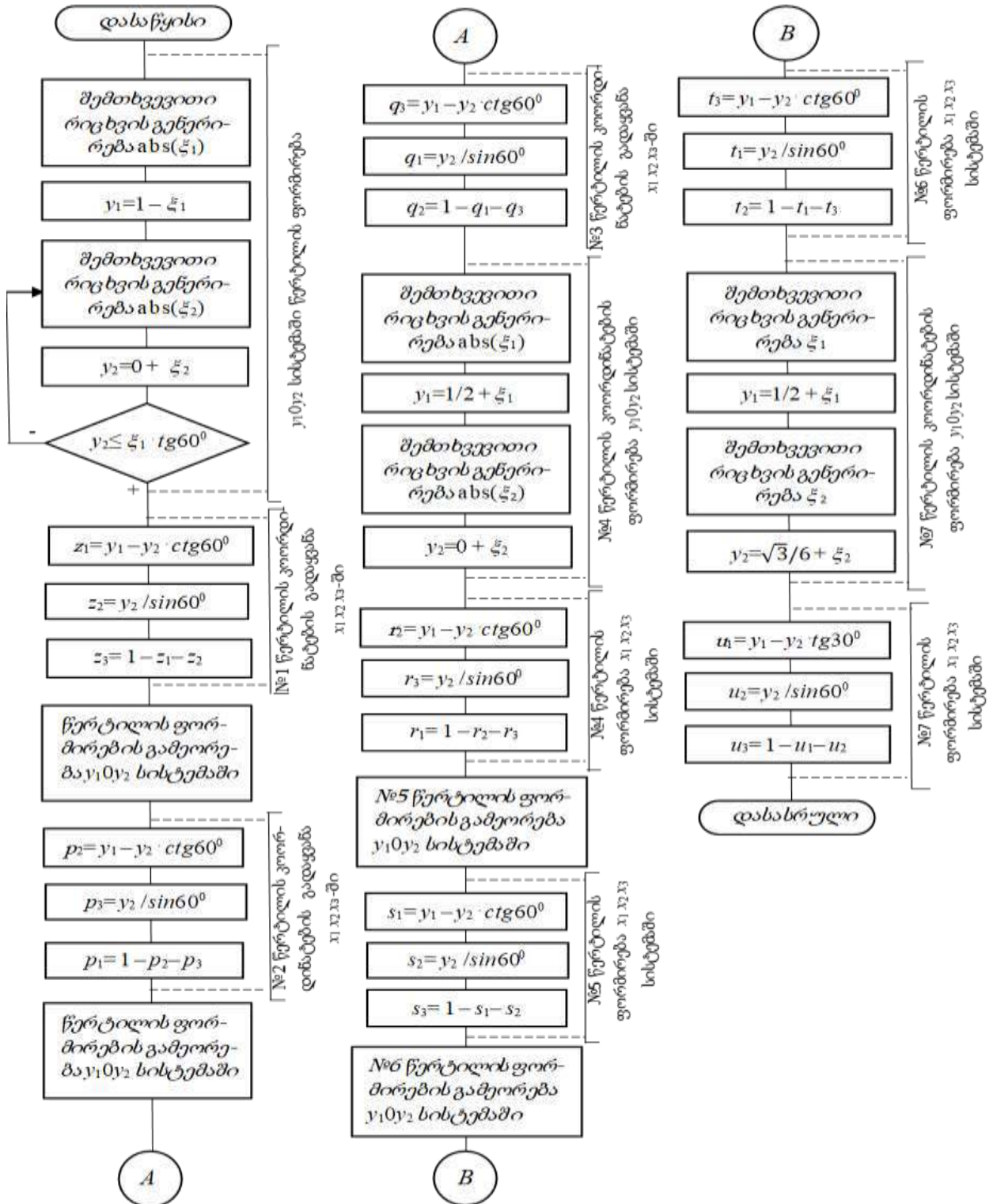
ნახ.2. ექსპერიმენტული შეცდომის პირობებში სამკომპონენტური სიმპლექს-გოსოსური გეგმის არასრული კუბური მოდელის კოორდინატების გენერირების ალგორითმი
