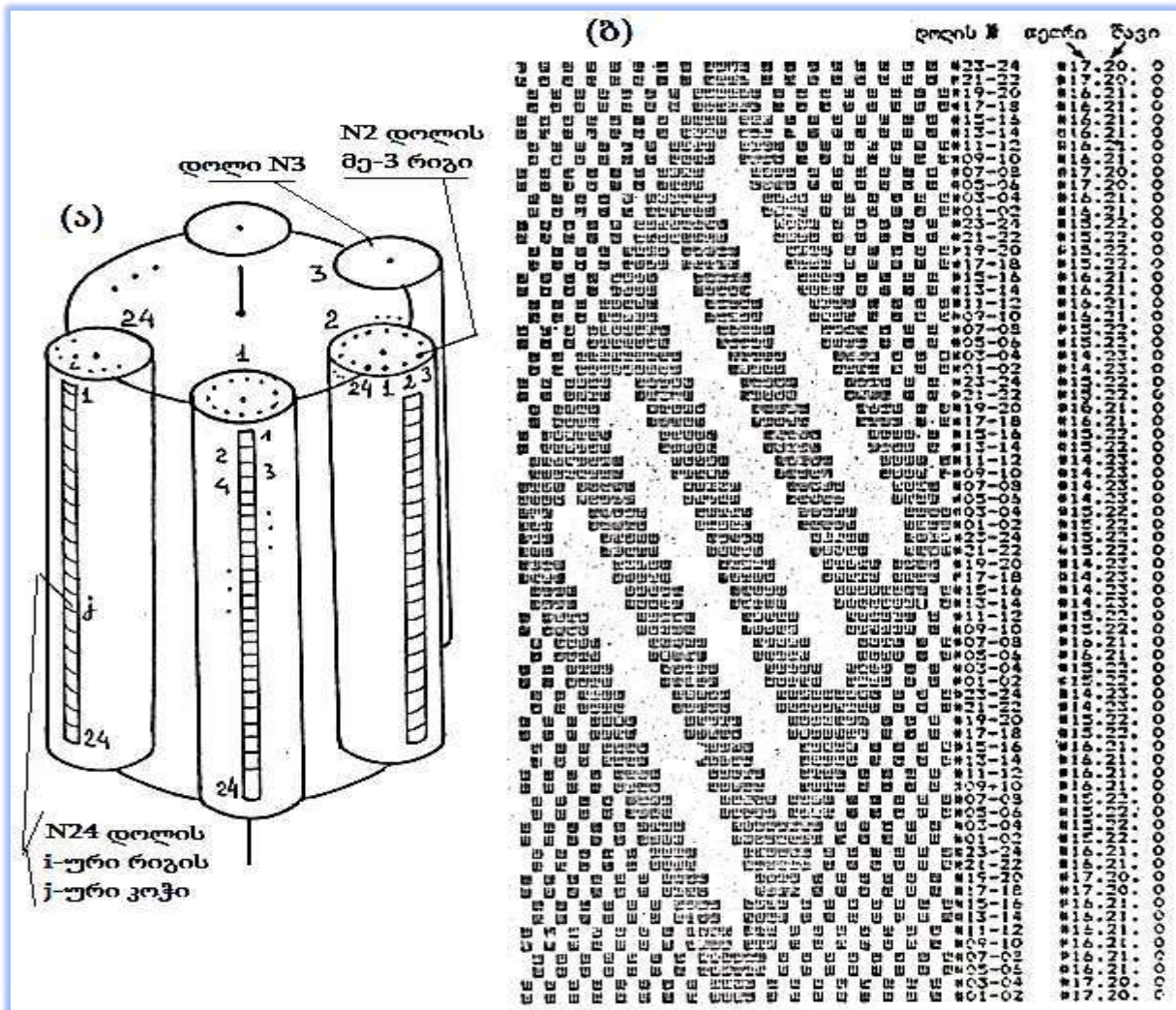
ნახ.4. მრგვალსაქსოვი სისტემის ფრაგმენტი (ა) და ქსოვილის ესკიზის მაკეტი (ბ), აგებული Robotron 1715-ზე (1988)
