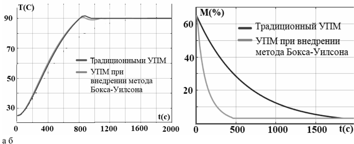
Рис 4. Сравнение работы традиционным УПМ и УПМ при внедрении метода Бокса-Уилсона для прогноза выхода объекта
