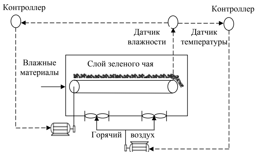
Рис. 1. Схема оцениваемой конвейерной сушилки
