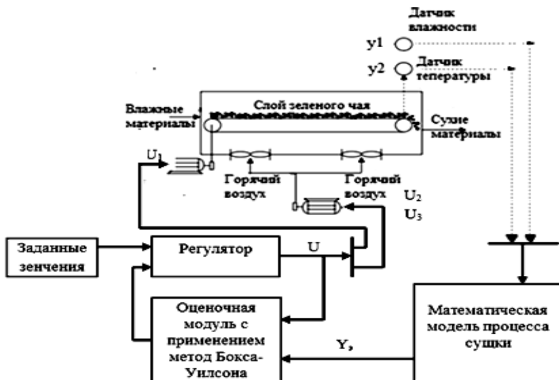
Рис. 2. Блок-схема системы управления с применением метода Бокса-Уилсона
