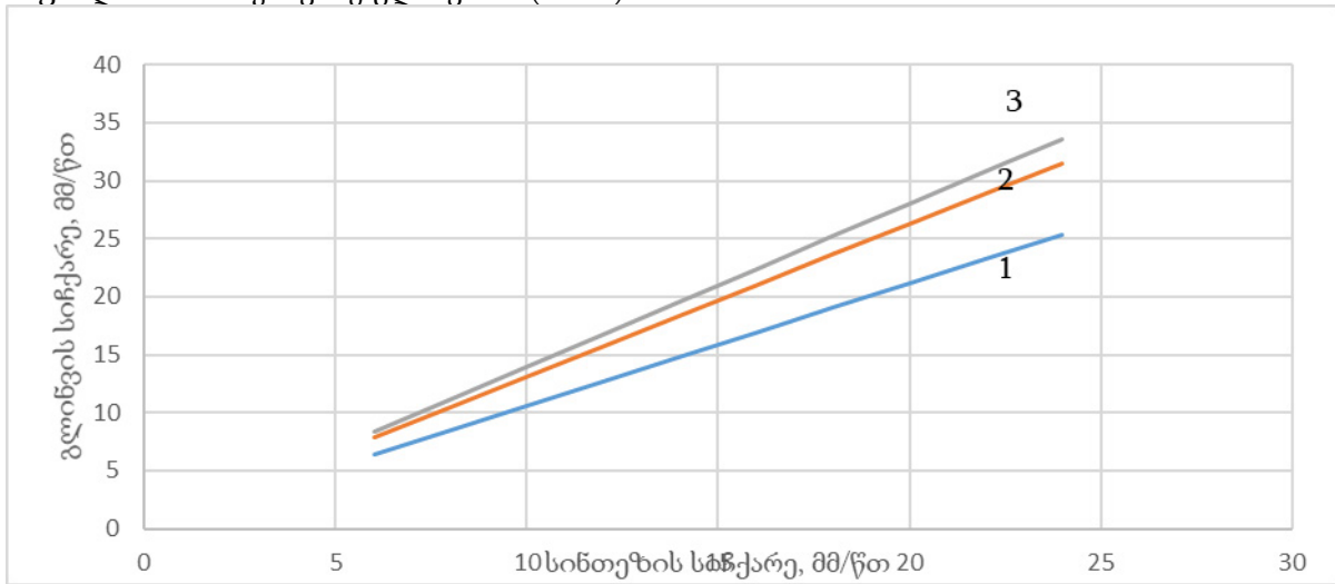
სურ.3. კორექტირებული გლინვის სიჩქარე, სინთეზის სხვადასხვა სიჩქარისგან დამოკიდებულებით ( \epsilon = 58,3\% ); 1- L=370მმ, 2- L=460მმ, 3- L=490მმ
