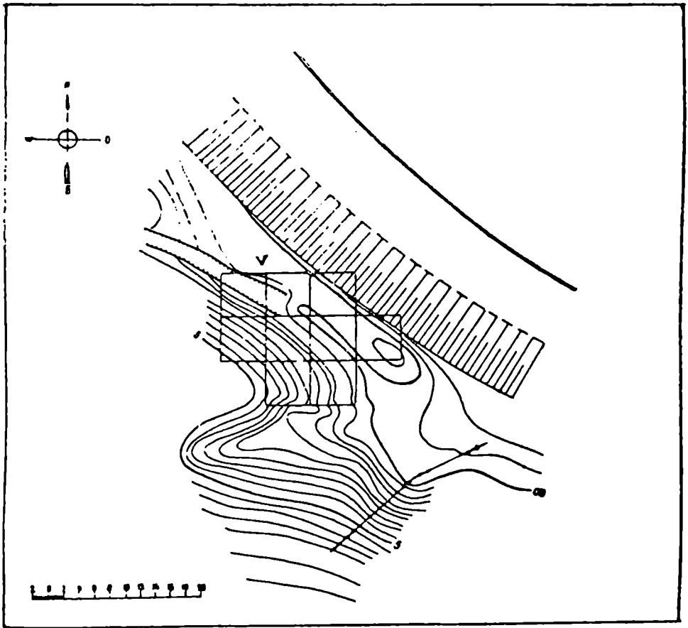
სურ. 18. კარსნისხევი. V ნაკვეთი. გეგმა
