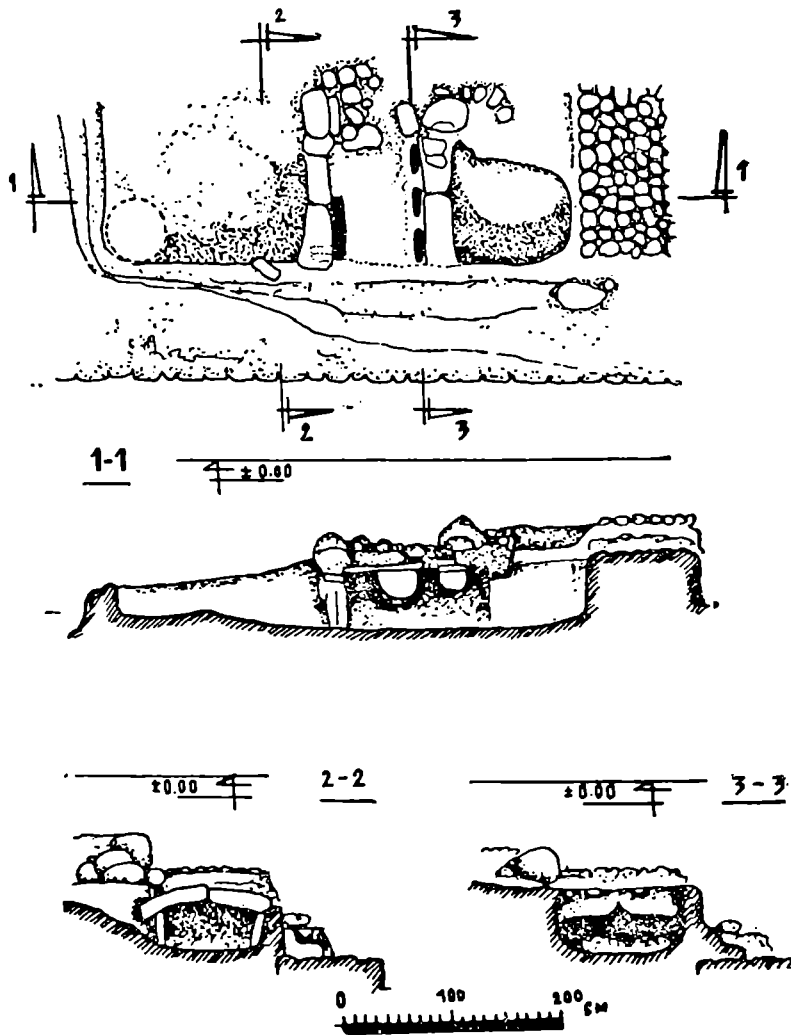
სურ. 10. კარსნისხევი. ქუჩა 4. ვეგმა, კრალეზი.
