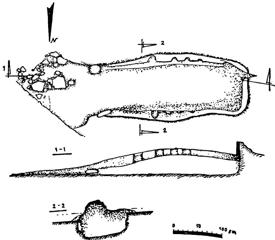
სურ. 9. კარსნისხევი. ქურა 3. გეგმა, კრილები
