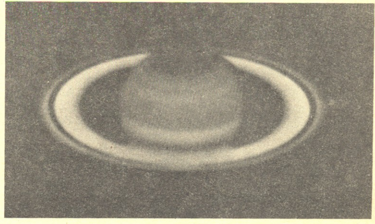
პლანეტა სატურნი, რგოლით
