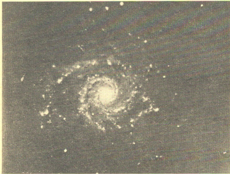
ჩვენს გალაქტიკის მსგავსი სპირალური გალაქტიკა № GC 628
