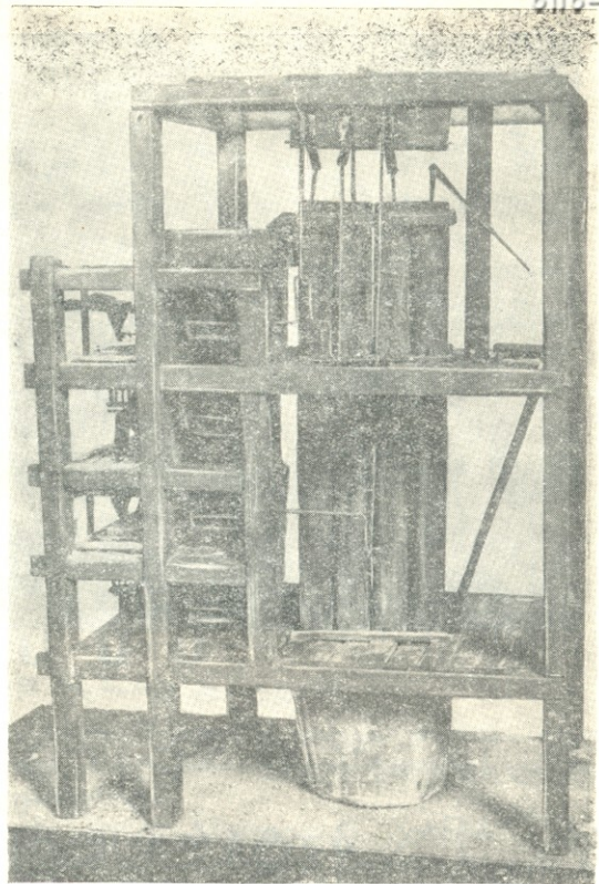
წისკვილის მაკეტი, შესრულებული დავით გურამიშვილის ნახაზის მიხედვით. (საიუბილეო გამოფენის მასალებიდან).
