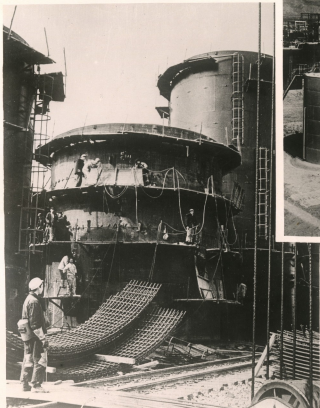
Строительство доменной печи № 2 Уханьского металлургического комбината.
