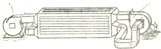
ჩაის საჭკნობი დანადგარი. 1-1. ვენტილატორები, 2. თაროებიანი ყუთი.
