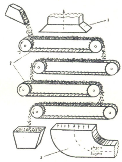
ჩაის სახმობი დანადგარი. 1. ცხელი ჰაერის გასასვლელი მილი. 2. ტრანსპორტიორები. 3. ცხელი ჰაერის შესასვლელი მილი.
