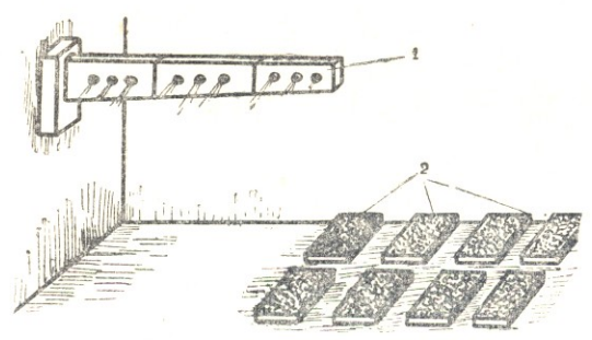
ჩაის საფერმენტაციო სააქრო. 1. პეკროტემბერი. 2. ყუთები დაგრებილი ჩაის ფოთლით.
