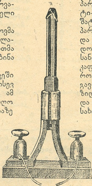
იაბლოჩკოვის სანთელი.
