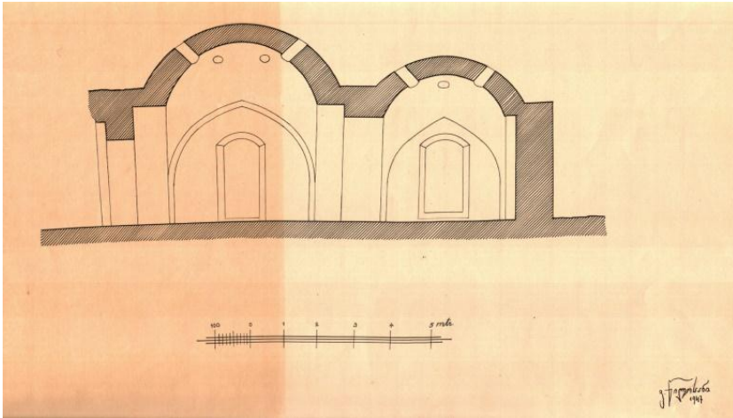
„ერეკლეს აბანო“, ნაგებობის ჭრილი. არქიტ. ვ. წილოსანი, 1947 წ. 1
