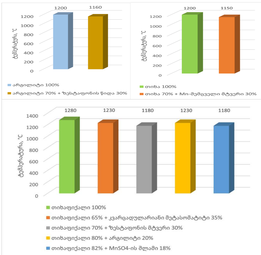
სურათი. 13 დანამატების გავლენა თიხოვანი ქანების აფუების ტემპერატურაზე
