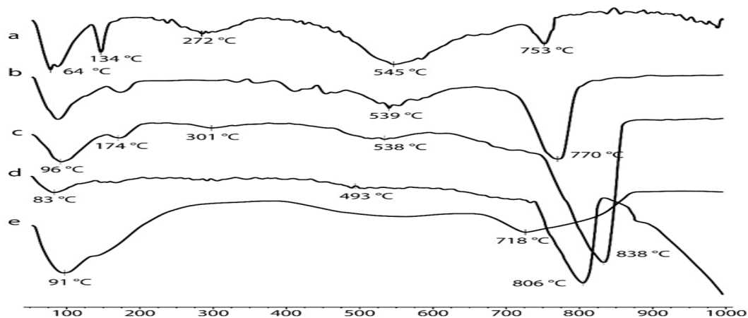
სურათი 2. თიხოვანი ქანების DTG მრუდები
