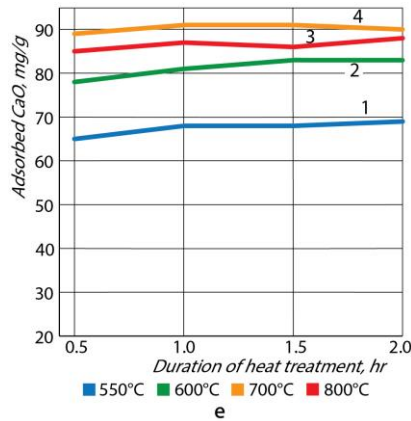
სურათი 4. ნაჯერი ხსნარიდან CaO-ს შთანთქმის კინეტიკა თიხოვანი ქანების მიერ
