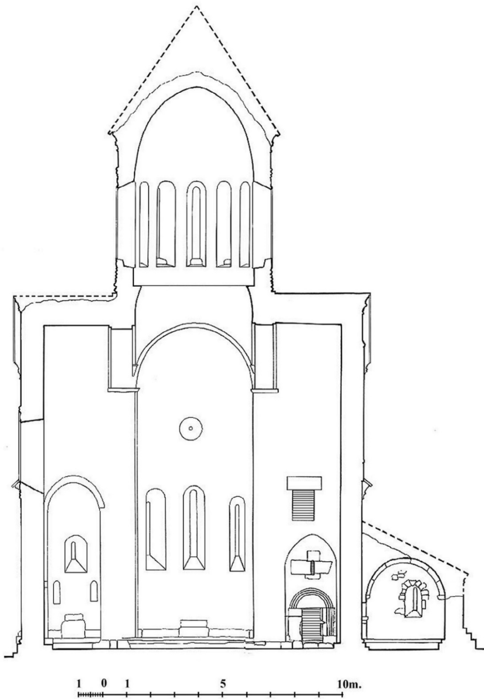
ნახ. 4. ჰუჯაბი. ჯვარგუმბათოვანი ტაძარი. განივი განაკვეთი ხედით აღმოსავლეთზე.
