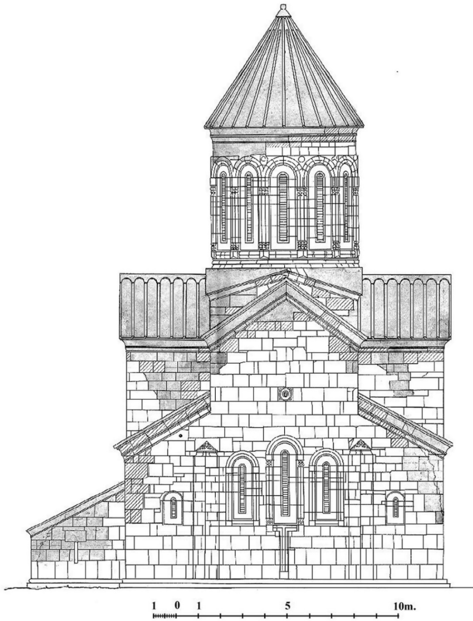
ნახ. 6. ჰუჯაბი. ჯვარგუმბათოვანი ტაძარი. აღმოსავლეთი ფასადი.
