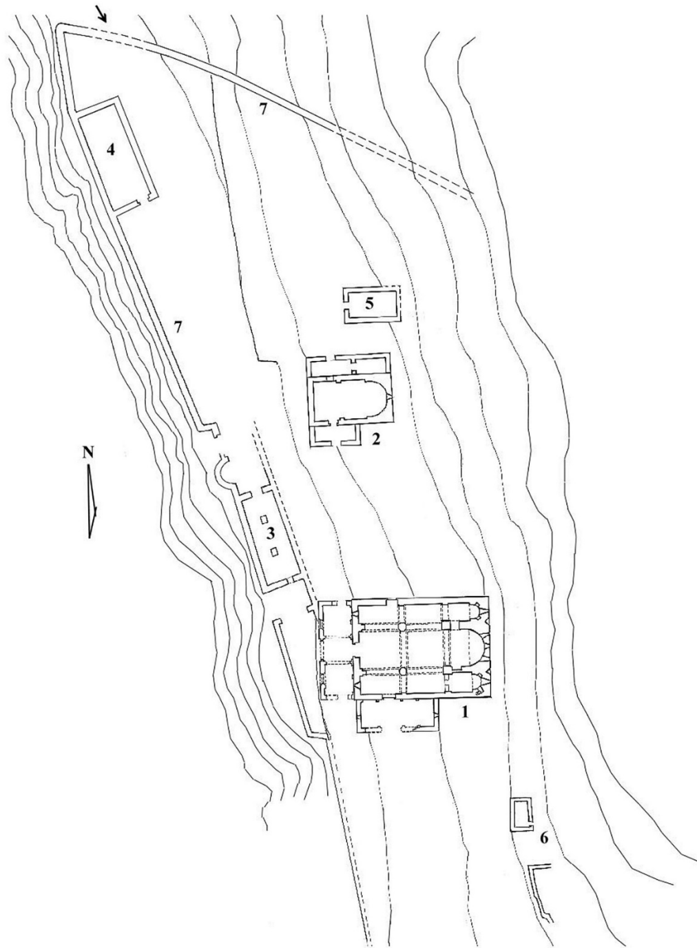
ნახ. 2. ჰუჯაბის სამონასტრო კომპლექსის გენგეგმა: 1. ჯვარგუმბათოვანი ეკლესია. XII–XIII სს–ის მიჯნა, XIII ს–ის პირველი მეოთხედი; 2. დარბაზული ეკლესია მინაშენებით. ადრექრისტიანული ხანა, ვიდრე X ს–მდე; 3. სატრაპეზო, მრგვალი კომპოზით და შესასვლელით(?); 4. სამონასტრო ნაგებობა; 5. მცირე ეკლესია (?) 6. სენაკი (?); 7. გალავანი.
