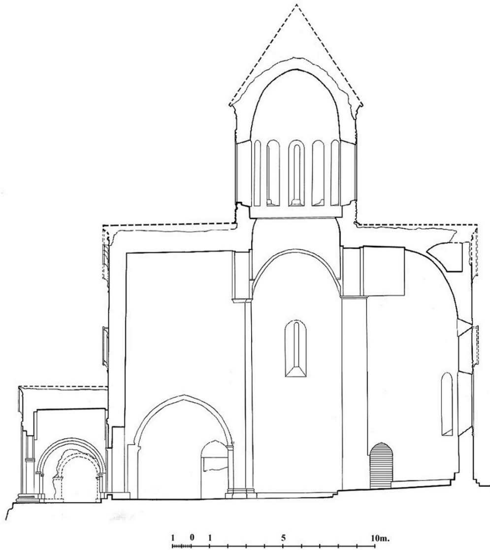
ნახ. 5. ჰუჯაბი. ჯვარგუმბათოვანი ტაძარი. სიგრძივი განაკვეთი ხედით ჩრდილოეთზე.
