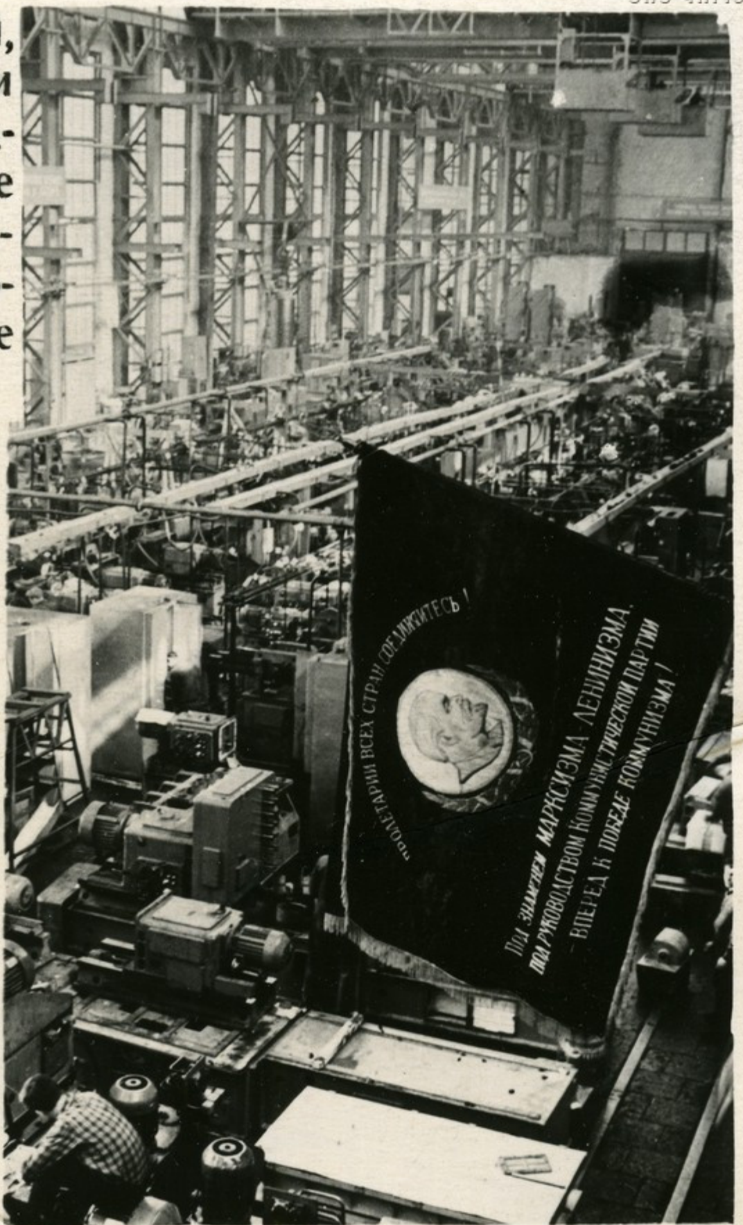
В сборочном цехе станкостроительного завода имени Серго Орджоникидзе смонтирована система автоматических линий для обработки головок цилиндров двигателей.
