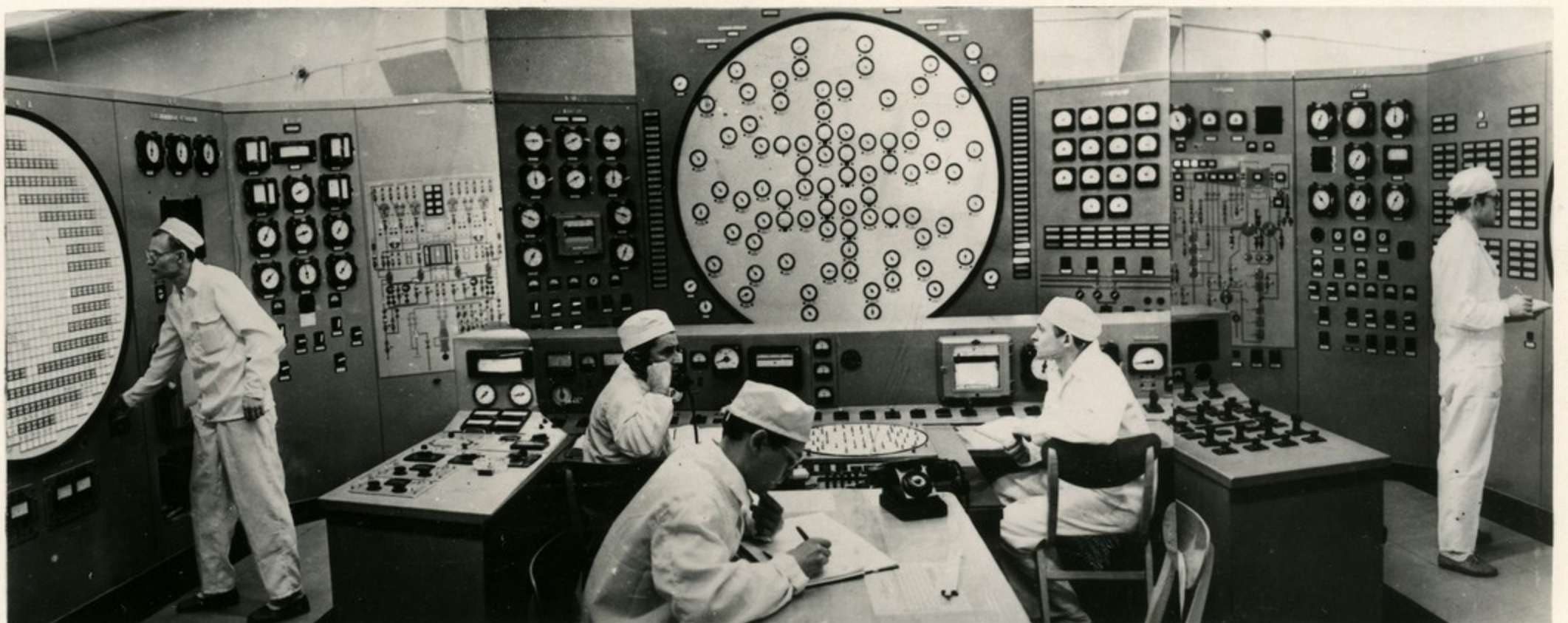
Свердловская область. У блочного щита управления Белоярской атомной электростанции имени И. В. Курчатова.
