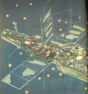
1. კოსმონავტი ილმინატორიდან დანტერის ფედიმონა. 2. კოსმონავტი ფეხ ცენტრალურ სამართავ პულტთან. 3. ფოტოაპარატი. 4. სასმელი წყლის მარაგი. 5. ზომილდე „სოიუზიდან“ „სალუბ-ში“ გადახედა. 6. ზომილდე „სოიუზის“ ორბიტალური განყოფილება. 7. შინს ზატარეები. 8. ფასაინებული აფილი. 9. ვენტლატორი. 10. რაბიტული ძრავები. 11. ასტენები, 12. ფედიმონაზე დანამები ზომილდე „სოიუზი“. 13. „სალუბთან“ შეპირაბირებული კოსმონავტი ზომილდე „სოიუზი“. 14. საცეპის მარაგი.
