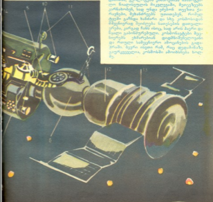
1. კოსმონავტი ილმინატორიდან დანტერის ფედიმონა. 2. კოსმონავტი ფეხ ცენტრალურ სამართავ პულტთან. 3. ფოტოაპარატი. 4. სასმელი წყლის მარაგი. 5. ზომილდე „სოიუზიდან“ „სალუბ-ში“ გადახედა. 6. ზომილდე „სოიუზის“ ორბიტალური განყოფილება. 7. შინს ზატარეები. 8. ფასაინებული აფილი. 9. ვენტლატორი. 10. რაბიტული ძრავები. 11. ასტენები, 12. ფედიმონაზე დანამები ზომილდე „სოიუზი“. 13. „სალუბთან“ შეპირაბირებული კოსმონავტი ზომილდე „სოიუზი“. 14. საცეპის მარაგი.
