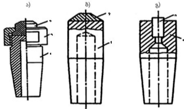
ნახ. 1. ელექტროდები მუშა ნაწილით სხვადასხვა ლითონისაგან.
