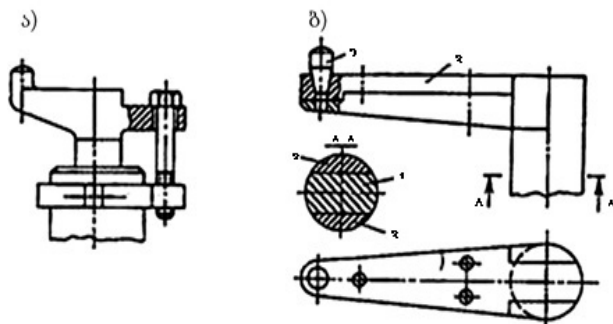
ნახ. 4. ელექტროდები, რომლებიც აღიქვამენ გალუნვის მაღალ მომენტს: ა – ელექტროდსაჭერის მიმაგრებით გარე ზედაპირზე; ბ – არმირებული ელექტროდი: 1 – ფოლადის კონსოლი; 2 – ელექტროდი; 3 – დენმიმყვანი ნერტილოვანი შედუღების დროს უმეტეს შემთხვევაში გამოიყენება ელექტროდების
