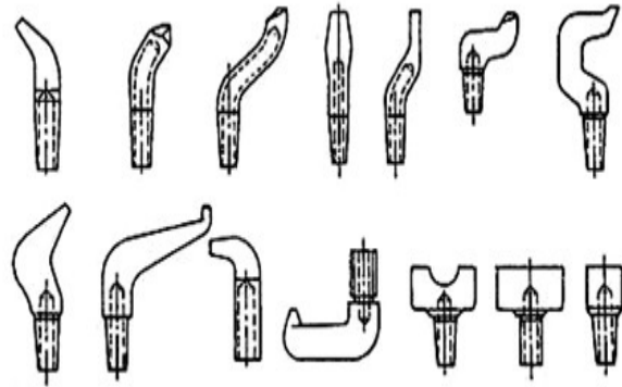
ნახ. 2. ფიგურული ელექტროდების სხვადასხვა ტიპები
