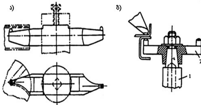
ნახ. 6. მრავალპოზიციური გადაყენებითი (ა) და ზედაპირული (ბ) ელექტროდები: 1 – ელექტროდდამჭერი; 2 – ელექტროდი
