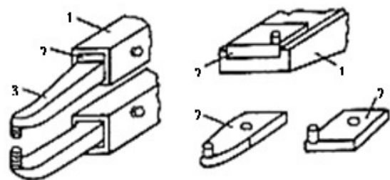
ნახ. 5. ელექტროდების დამაგრების ხერხები: 1. ელექტროდდამჭერი; 2. სამაგრი; 3. ელექტროდის ტანი
