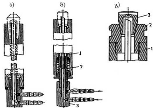
ნახ. 7. სწორი ელექტროდდამჭერები: ა – ნორმალური; ბ – გამომგდებითი; გ – ცვლადი მილისით. 1. გამომგდები; 2. ზამბარა; 3. ელექტროდი.
