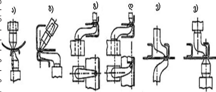
ნახ. 3. ფიგურული ელექტროდების გამოყენების ნიმუშები.
