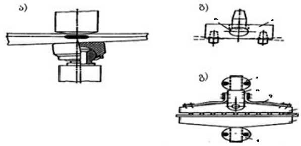
ნახ. 9. თვითდაყენებადი ელექტროდები და თავები:
