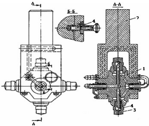
ნახ. 8. საბრუნო ელექტროდური თავი: 1 – საბრუნო ელექტროდდამჭერი; 2 – კორპუსი; 3 – ელექტროდი; 4 – საჭერი.
