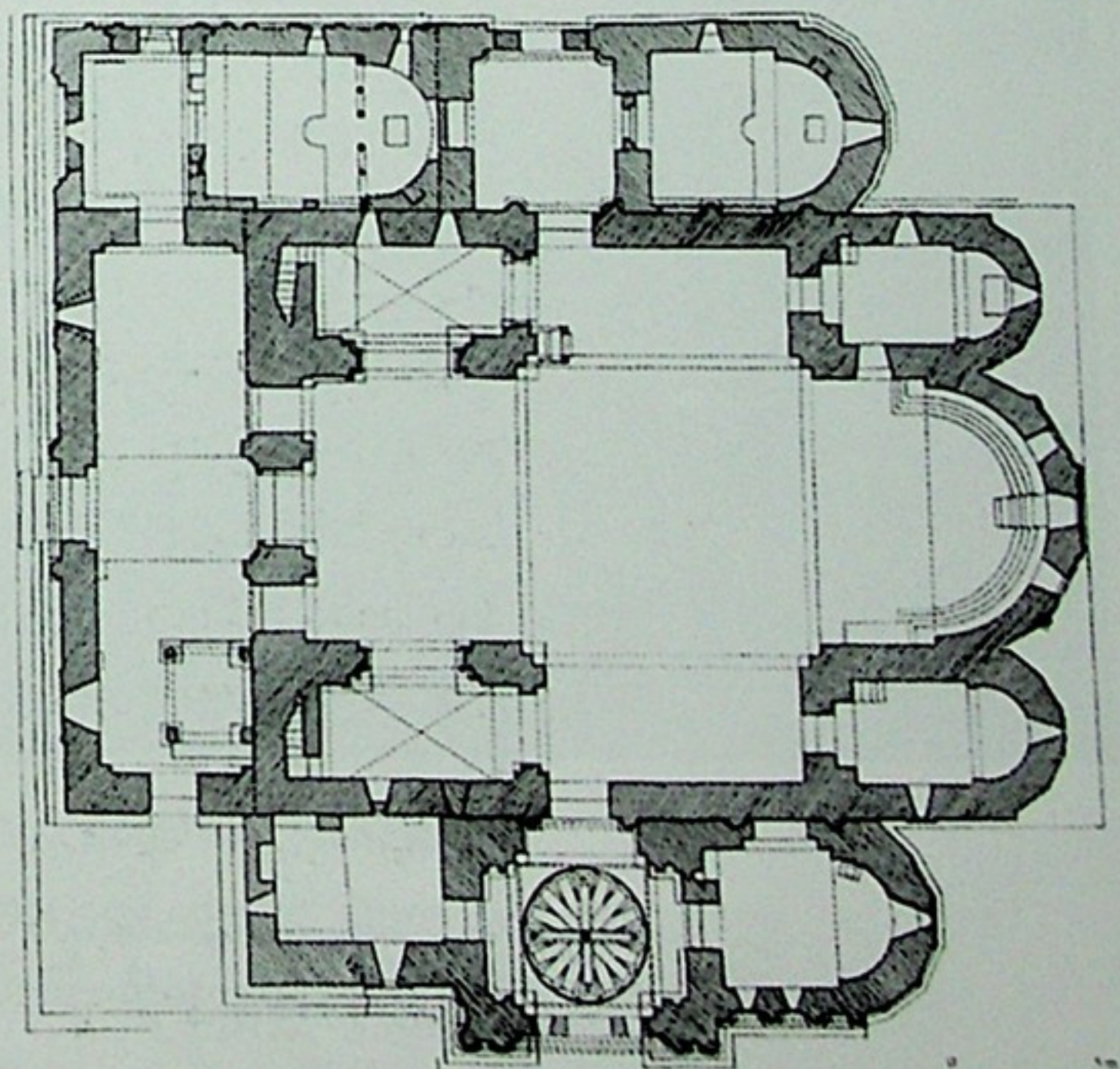
ღვთისმშობლის ტაძრის გეგმა
