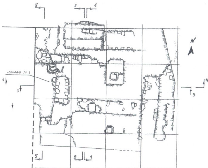
ნახ. 1. ეკლესიის აღმოსავლეთით მდებარე ტერიტორიის გათხრების გეგმა.
