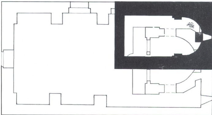
ნახ. 1. V-VII სს. ეკლესიის გეგმა.
