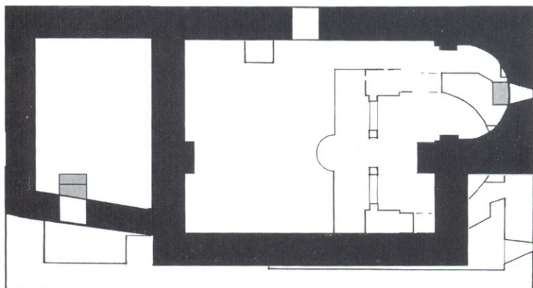
ნახ. 2. XII-XIV სს. კელესიის გეგმა.
