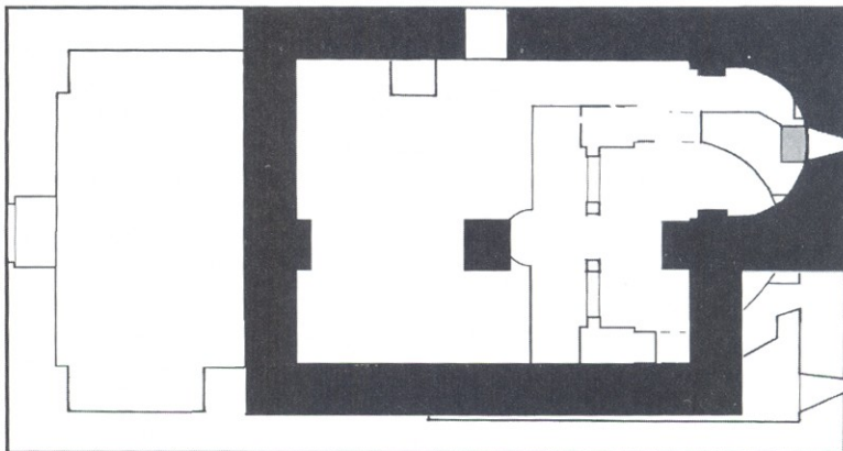
ნახ. 1. VIII-IX სს. კელესიის გეგმა.
