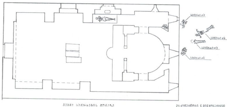
ნახ. 1 ეკლესიის ცენტრალურ ნაწილში გამოვლენილი სამი სამარხის ქვის სახურავის ფილები, გეგმა.
