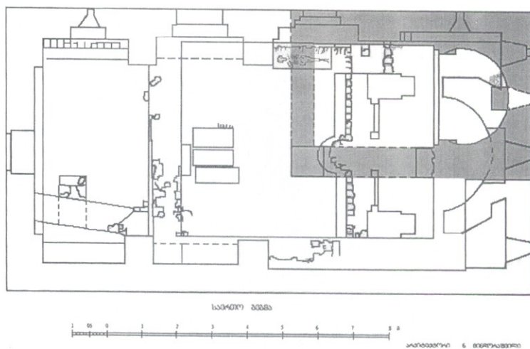
ნახ. 2. ეკლესიის საერთო გეგმა, გათხრების შემდეგ.
