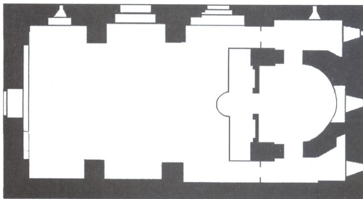
ნახ. 1. ეკლესიის გეგმა გათხრების შემდეგ.
