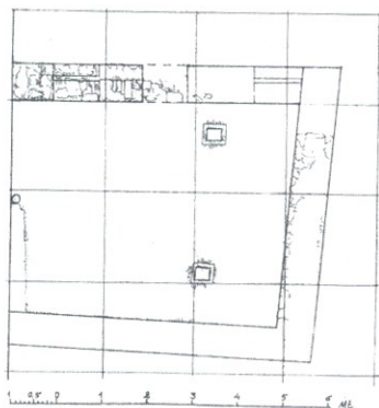
ნახ. 2. ეკლესიის აღმოსავლეთით მდებარე გათხრილი ტერიტორიის გეგმა და დარბაზული ტიპის ბანური სახლის რეკონსტრუქციის ცდა.
