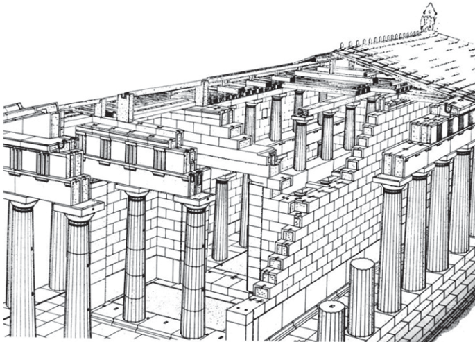
დორიული ორდერის კონსტრუქციული სისტემა
