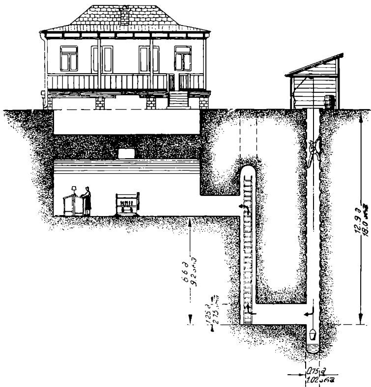
ავლაბრის ფარული ბოლშევიკური სტამბის ქების მოწყობილობის სქემა
