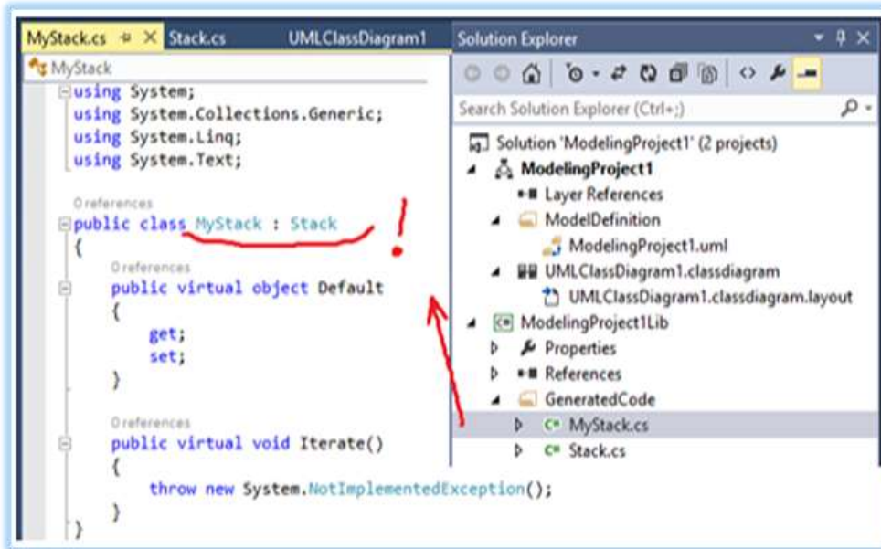
ნახ.19. კლასიდან გენერირებული Stack.cs კოდი
