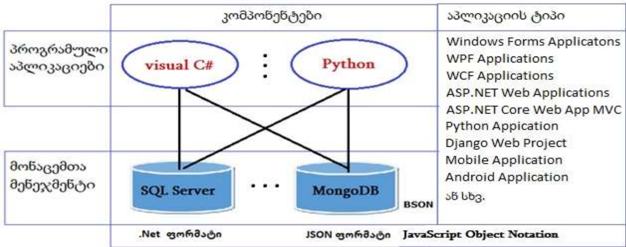
ნახ.27. აპლიკაციის ტიპები და კომპონენტები
