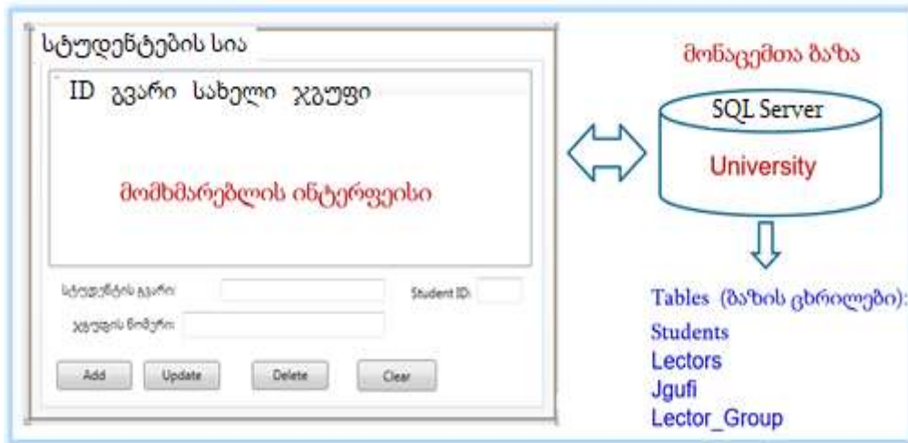
ნახ.28. პროგრამული აპლიკაციის ზოგადი სქემა
