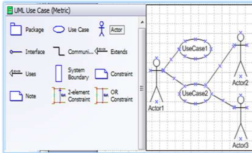
ნახ.4. UseCase დიაგრამის აგების ინტერფეისი (Visual Studio 2015)
