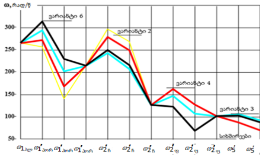
ნახ. 4. სიხშირეების განაწილება საგზაო სამოსის ფენებში
