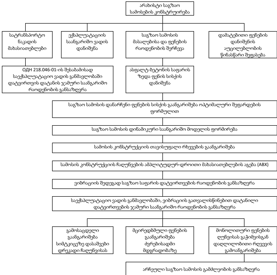
ნახ. 8. არახისტი საგზაო სამოსების კონსტრუქციის ბლოკ-სქემა, ვიბრაციული ფაქტორის გათვალისწინებით.
