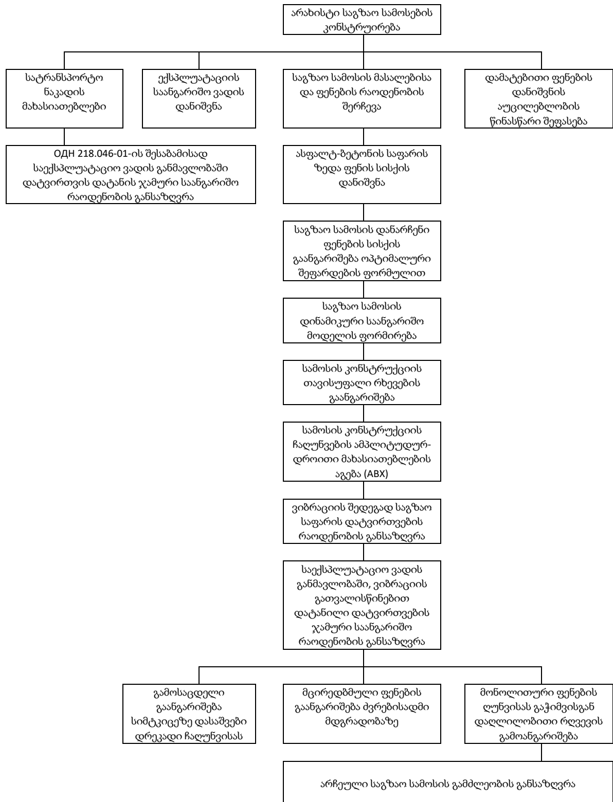
ნახ.22. არახისტი საგზაო სამოსების კონსტრუქციების ბლოკ-სქემა, ვიბრაციული ფაქტორის გათვალისწინებით.
