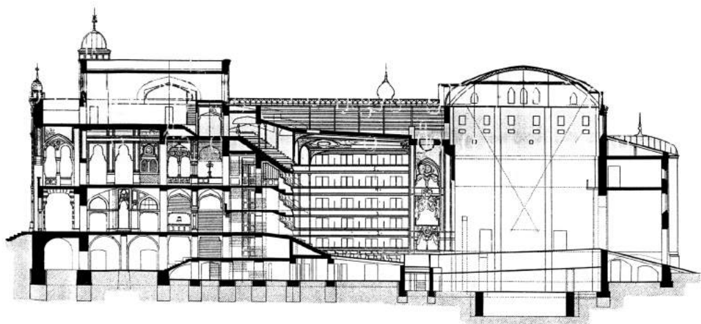
26. სახაზინო თეატრი. ჭრილი. არქიტექტორი ვ.შრამტაძე. 1880 წ.
