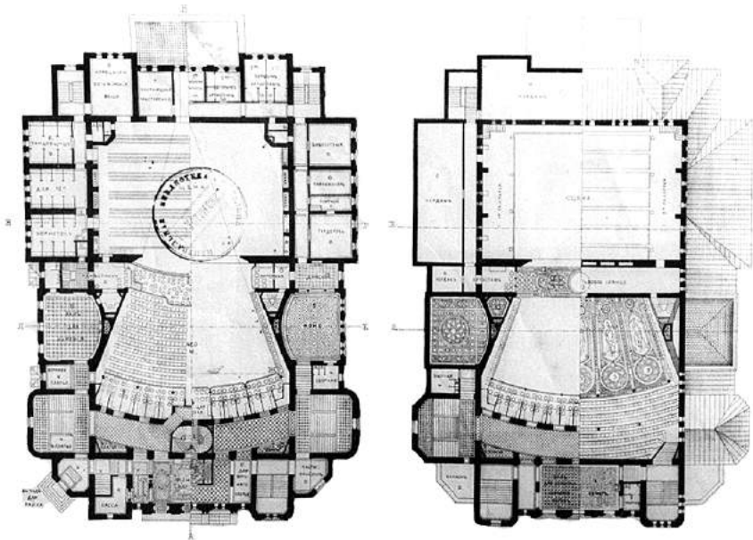
25. სახანინემ თეატრის საკონსტრუქციო პროექტი. არქიტექტორი ვ. ვერბოვი. 1877 წ.
