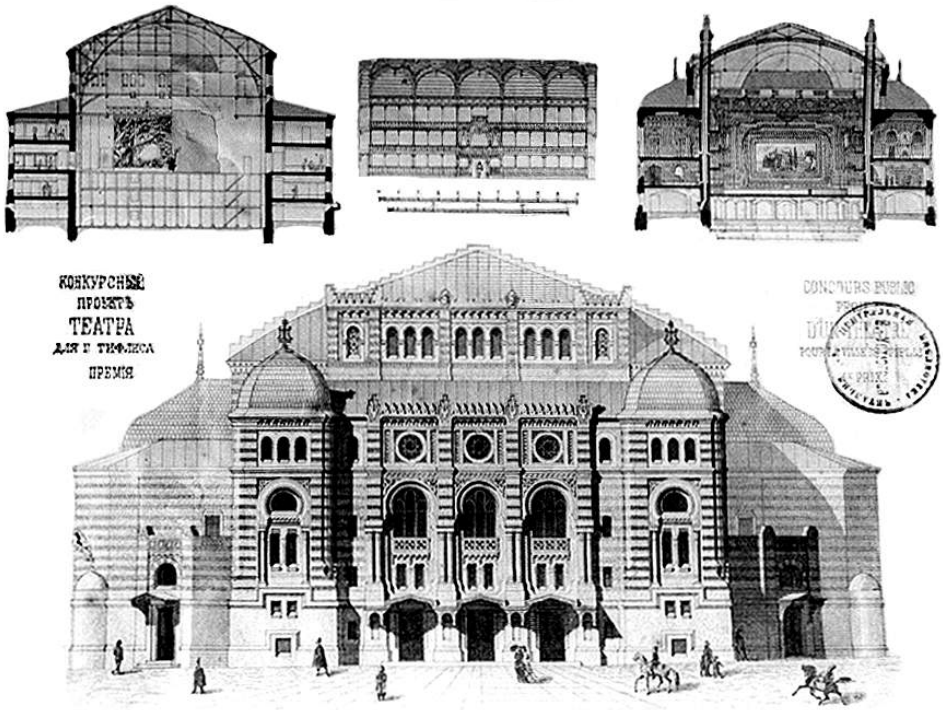
24. სახანინემ თეატრის საკონსტრუქციო პროექტი. არქიტექტორი ვ. ვერბოვი. 1877 წ.
