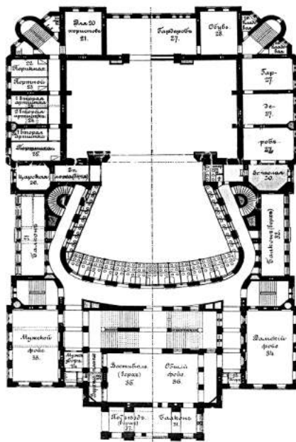
27. სახაზინო თეატრის პროექტი. არქიტექტორი ვ.შრამტაძე. 1880 წ.
