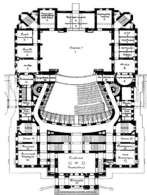
27. სახაზინო თეატრის პროექტი. არქიტექტორი ვ.შრამტაძე. 1880 წ.
