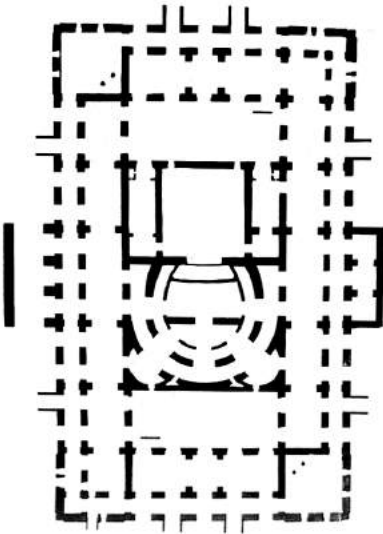
19.3. სარღვისა და ჯედა სართულის გეგმები.
