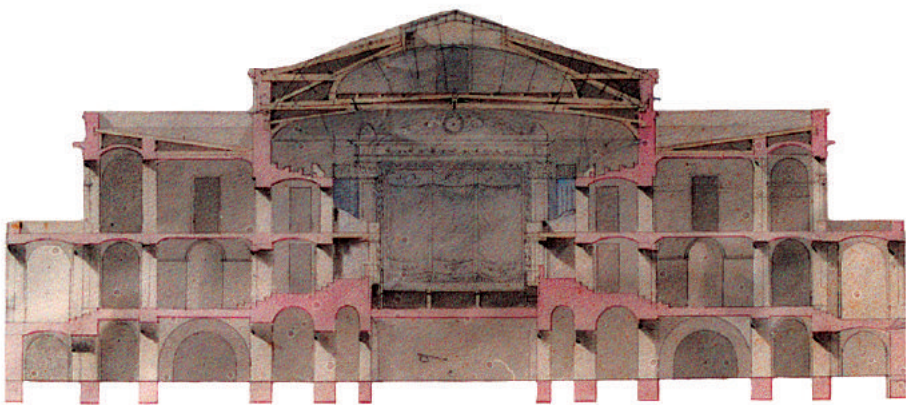
2. ქარვასლის თეატრის ბანივი ჭრილი. ჯ. სკუდნიერი. 1846-1851 წწ.
