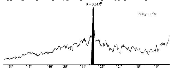
სურ. 7. №3 მძივის რენტგენოფაზური ანალიზის რენტგენოგრამა
