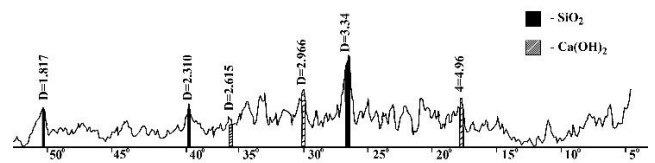
სურ. 3. № 2 მძივის რენტგენოფაზური ანალიზის რენტგენოგრამა
