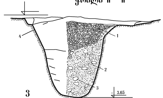
ქროლი II - II
