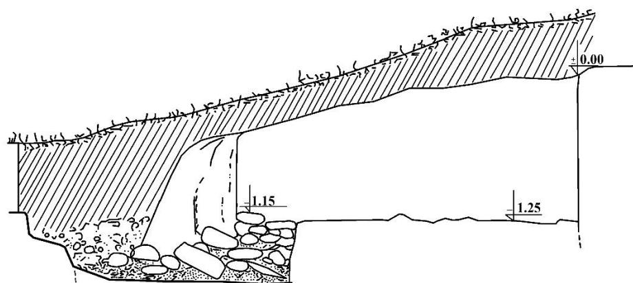
ჭრილი I - I
