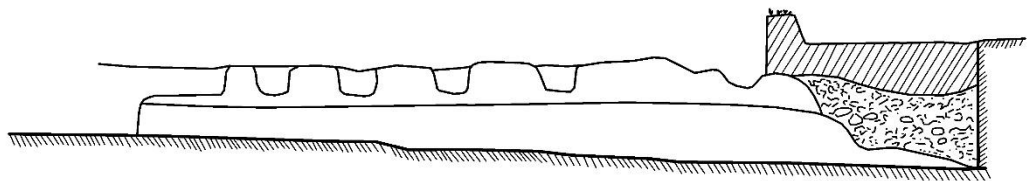
ჭრილი IV - IV
