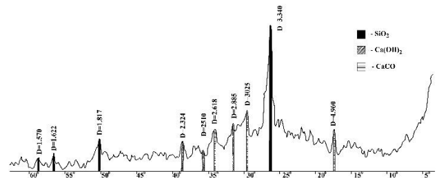
სურ. 14. № 12 მძივის რენტგენოფაზური ანალიზის რენტგენოგრამა
