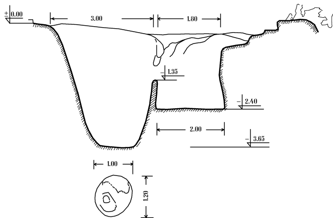
ჭრილი I - I
