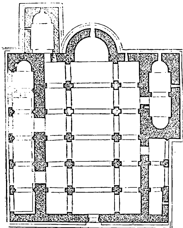
Рис. 1. План по обмеру арх. Цналы Габашвили 1936 года.
