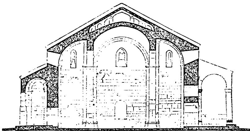
Рис. 5. Поперечный разрез с видом на восток.
