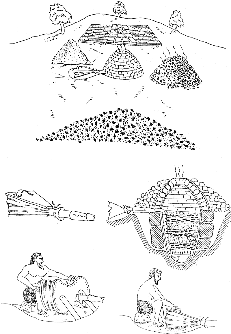
სურ. 1. ძველკოლხური რკინის სადნობი სახელოსნოს რეკონსტრუქცია. შესრულებულია ანზორ ჯაგელიძის მიერ
