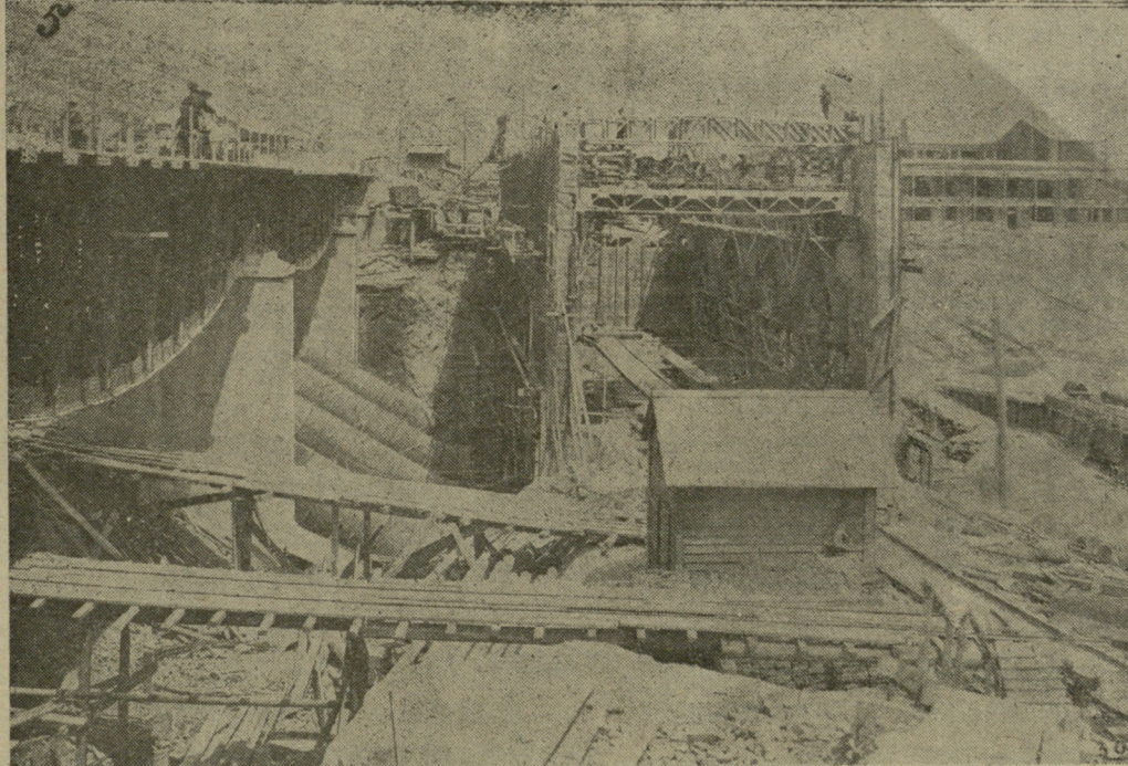
1. ჰიდრო-სადგურის და განმანაწილებელი სანმარტვლის შენობები, 2. მცხეთის ახალი ხიდი, რომელსაც ახლა აკეთებენ, 3. ჰიდრო-ელექტრონის სადგურის შენობა, 4. მთავარი სადგურის სახე ქვედა მხრიდან, 5. ვიალუკი, მწვევი მილები და ჰიდრო-ელექტრონის სადგურის შენობა. 6. ჰიდრო-ელექტრონის სადგურის გენერატორი.
