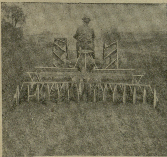
ტრაქტორი თევზებიან ფარცხით აოშებს ნიადაგს
