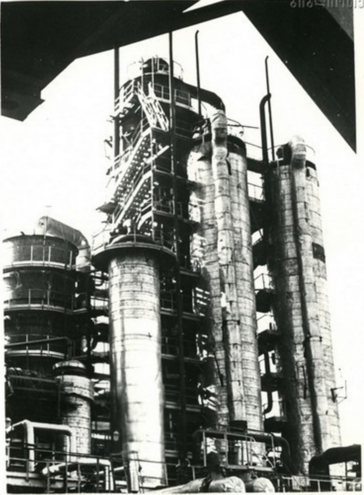
Аммиачное производство Руставского химкомбината
