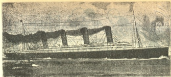
გემი „ტიტანიკი“.
