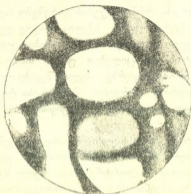
ვენერა.
