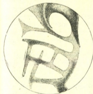
მერკური.
