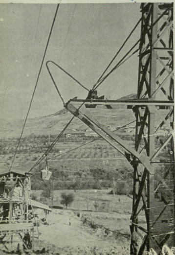
▲ ლიტონის საბაგირო გზის ტროლეიბან.
